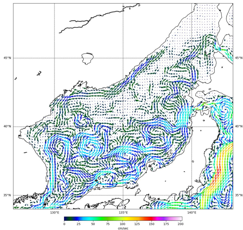
Рис. 3-2 Поверхностные течения Японского моря, 15 июля 2023 г.
