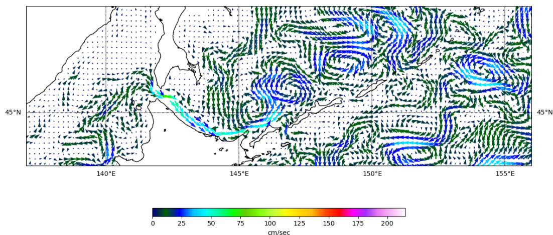
Рис. 3-7 Поверхностные течения, южная часть Охотского моря, 5 июля 2023 г.
