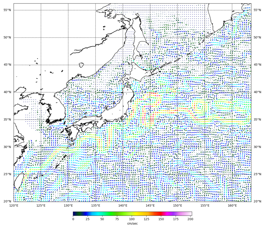
Рис. 3-5 Поверхностные течения западной части Тихого океана, 15 июля 2023 г.
