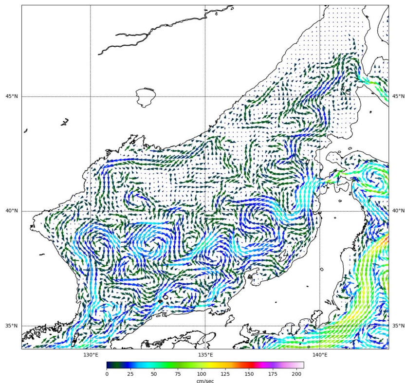
Рис. 3-3 Поверхностные течения Японского моря, 25 июля 2023 г.
