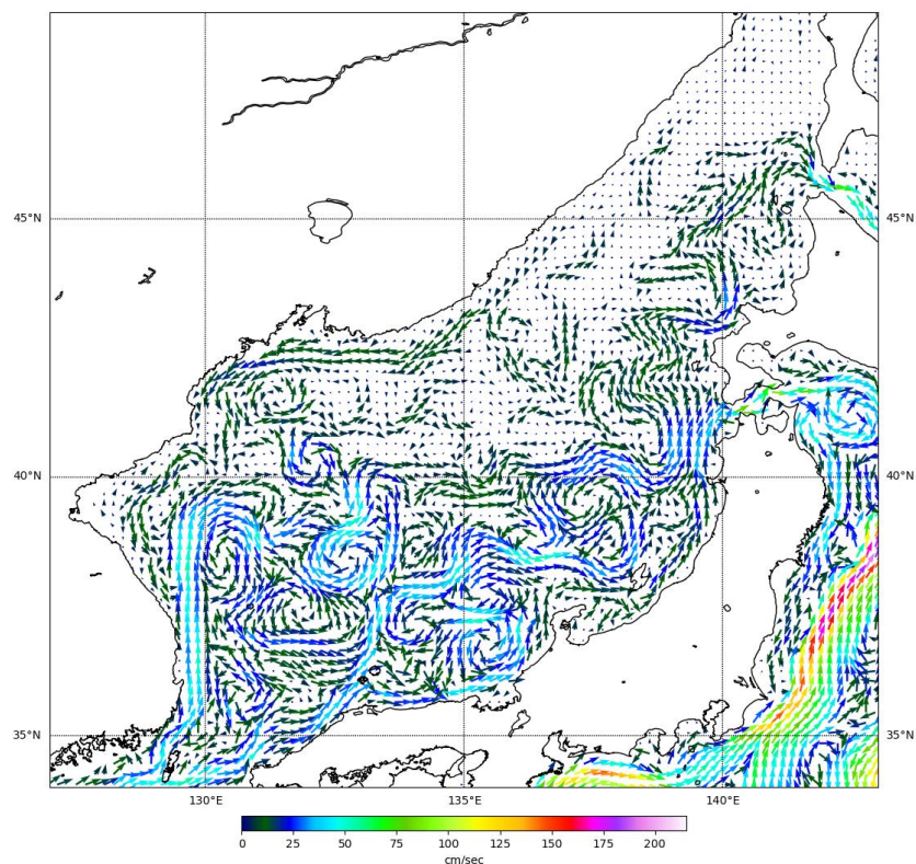
Рис. 3-1 Поверхностные течения Японского моря, 05 июля 2023 г.
