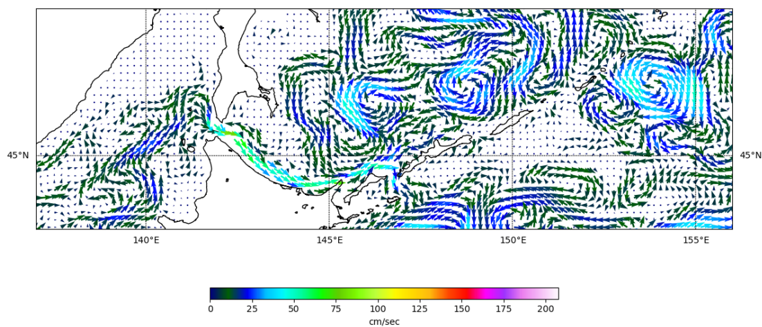
Рис. 3-9 Поверхностные течения, южная часть Охотского моря, 25 июля 2023 г.
