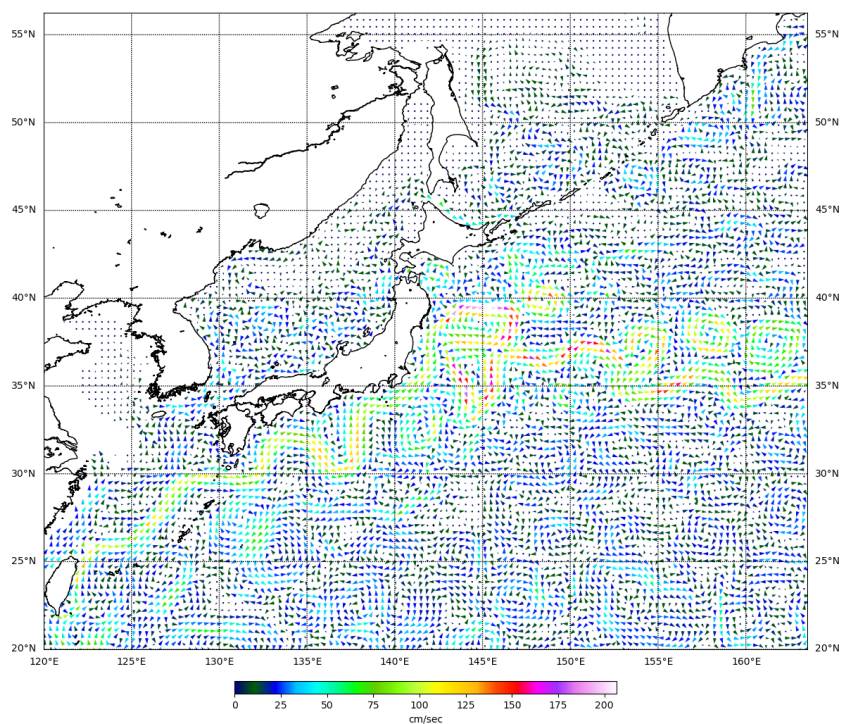
Рис. 3-6 Поверхностные течения западной части Тихого океана, 25 июля 2023 г.
