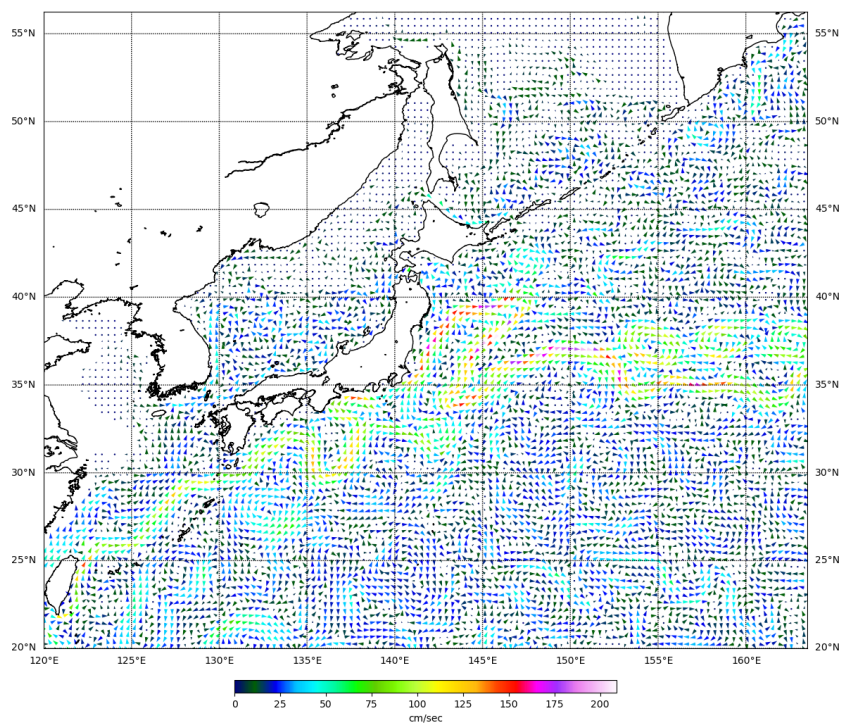
Рис. 3-4 Поверхностные течения западной части Тихого океана, 5 июля 2023 г.
