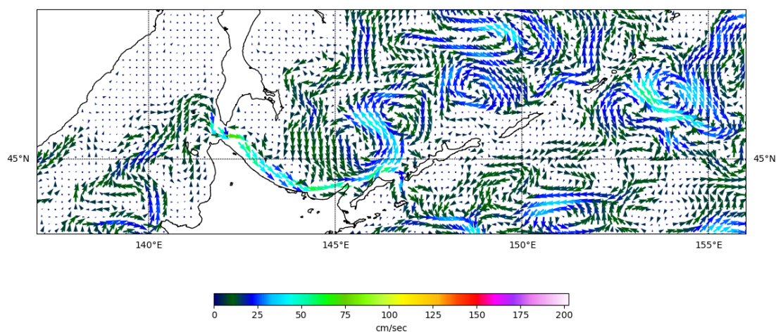
Рис. 3-8 Поверхностные течения, южная часть Охотского моря, 15 июля 2023 г.
