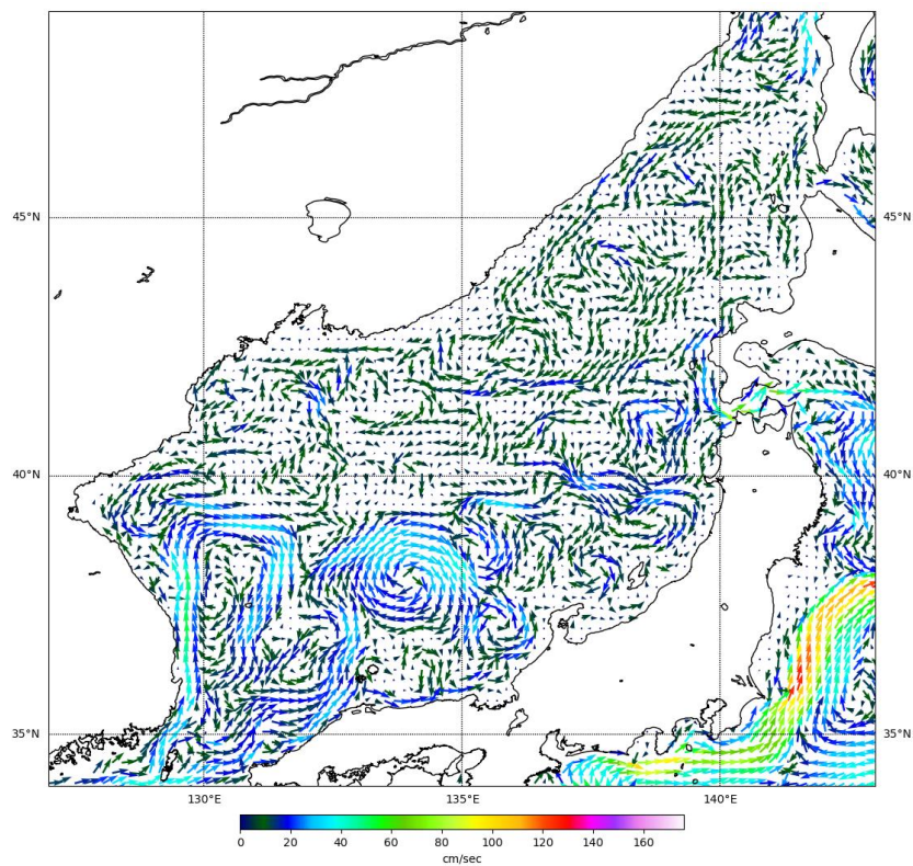
Рис. 3-3 Поверхностные течения Японского моря, 25 января 2023 г.
