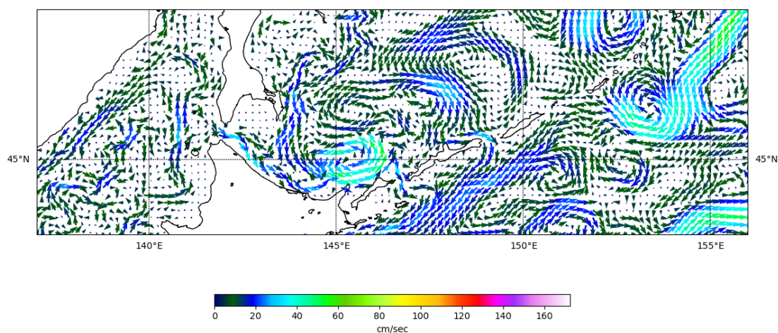
Рис. 3-8 Поверхностные течения, южная часть Охотского моря, 15 января 2023 г.
