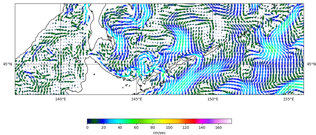
Рис. 3-9 Поверхностные течения, южная часть Охотского моря, 25 января 2023 г.
