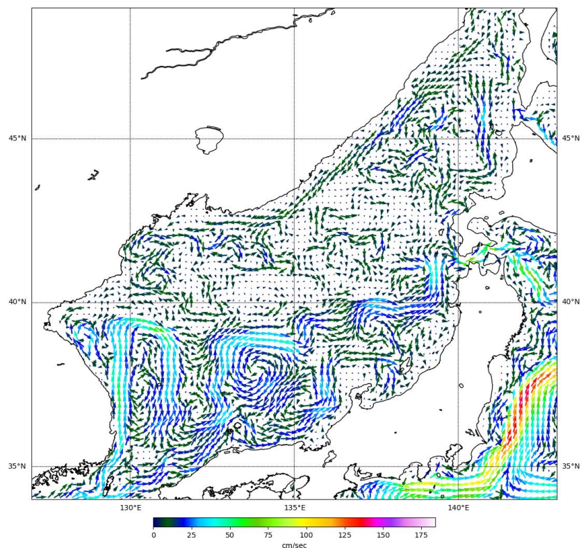
Рис. 3-1 Поверхностные течения Японского моря, 05 января 2023 г.
