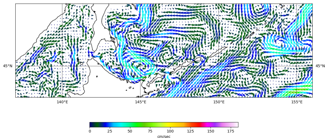
Рис. 3-7 Поверхностные течения, южная часть Охотского моря, 5 января 2023 г.
