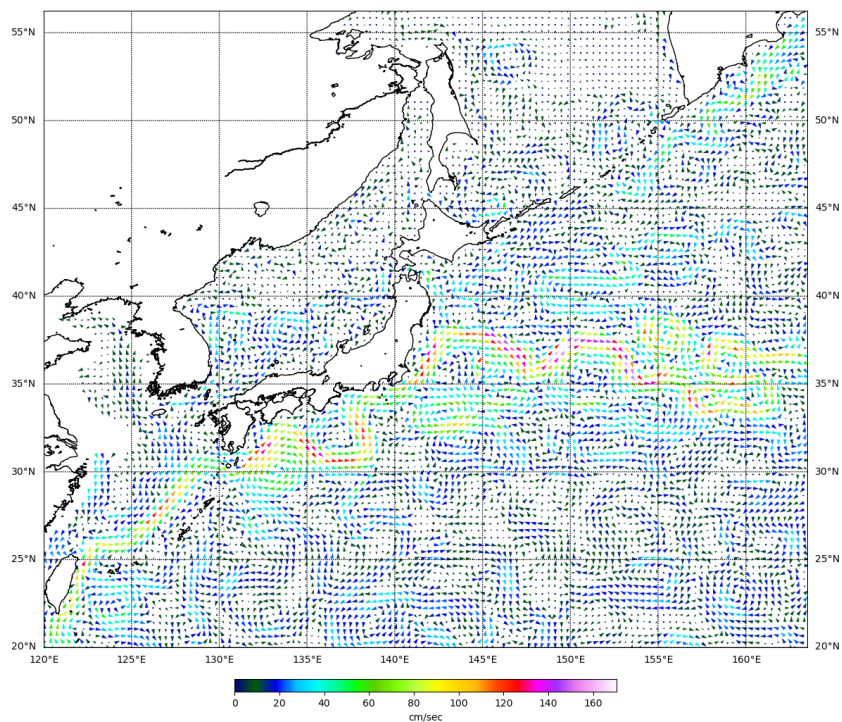
Рис. 3-5 Поверхностные течения западной части Тихого океана, 15 января 2023 г.
