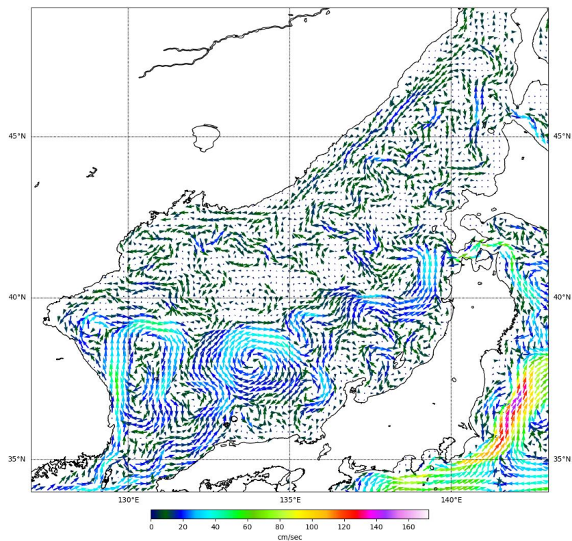
Рис. 3-2 Поверхностные течения Японского моря, 15 января 2023 г.
