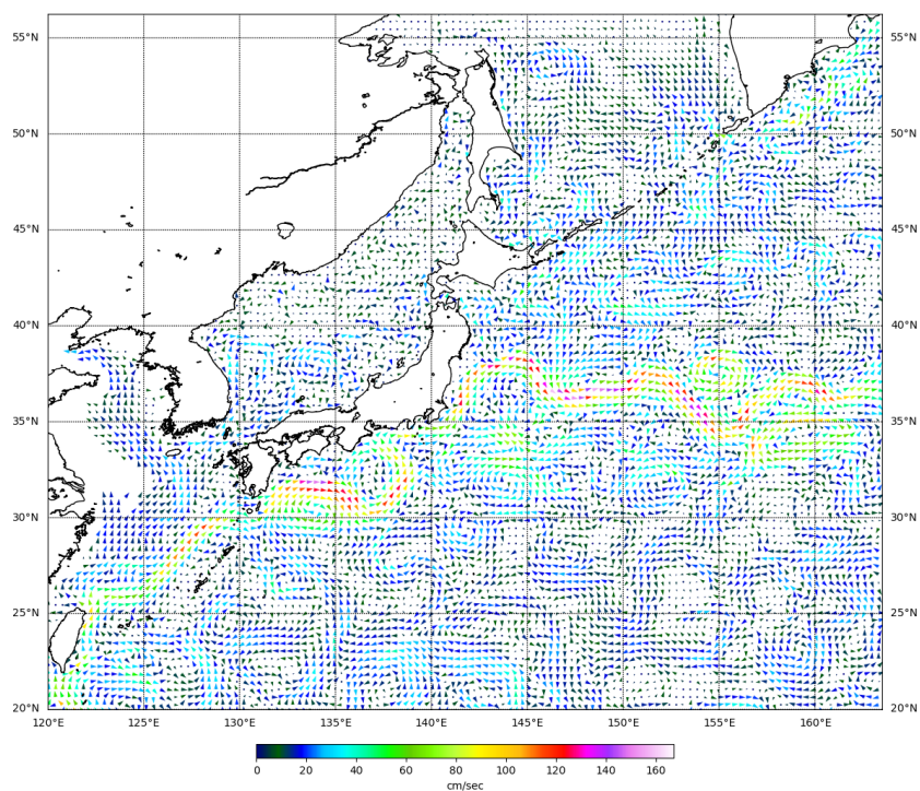
Рис. 3-6 Поверхностные течения западной части Тихого океана, 25 января 2023 г.
