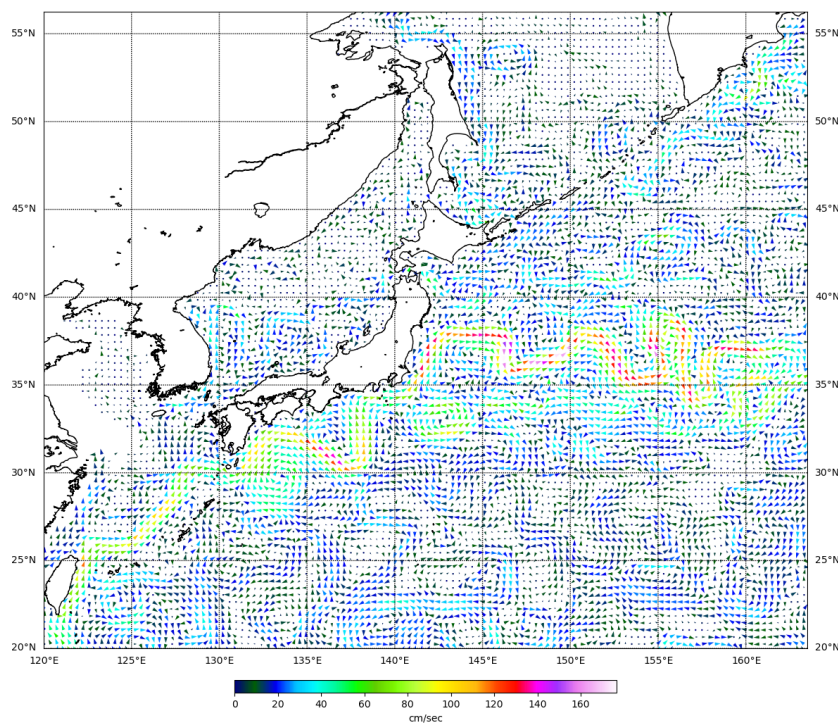
Рис. 3-4 Поверхностные течения западной части Тихого океана, 5 января 2023 г.
