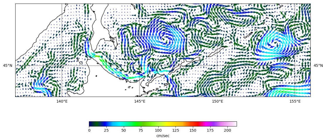
Рис. 3-9 Поверхностные течения, южная часть Охотского моря, 25 сентября 2022 г.
