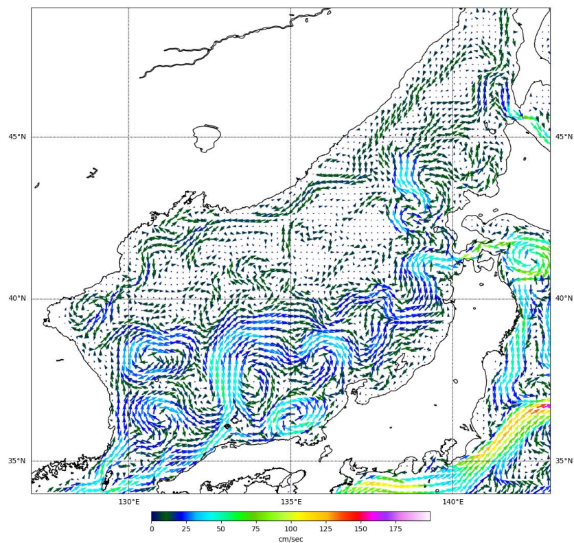
Рис. 3-2 Поверхностные течения Японского моря, 15 сентября 2022 г.
