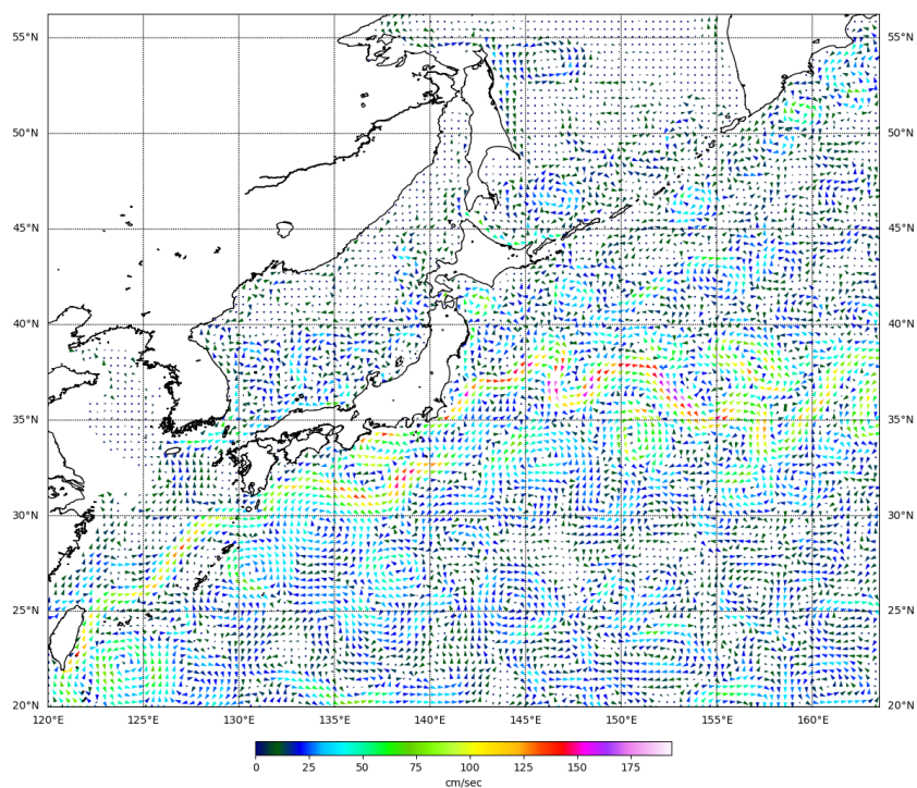
Рис. 3-6 Поверхностные течения западной части Тихого океана, 25 сентября 2022 г.
