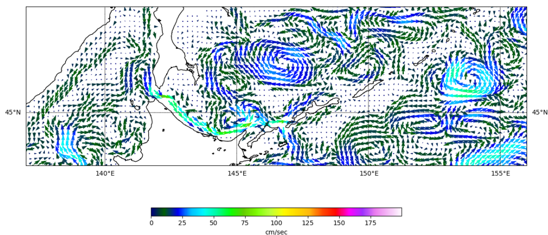
Рис. 3-8 Поверхностные течения, южная часть Охотского моря, 15 сентября 2022 г.
