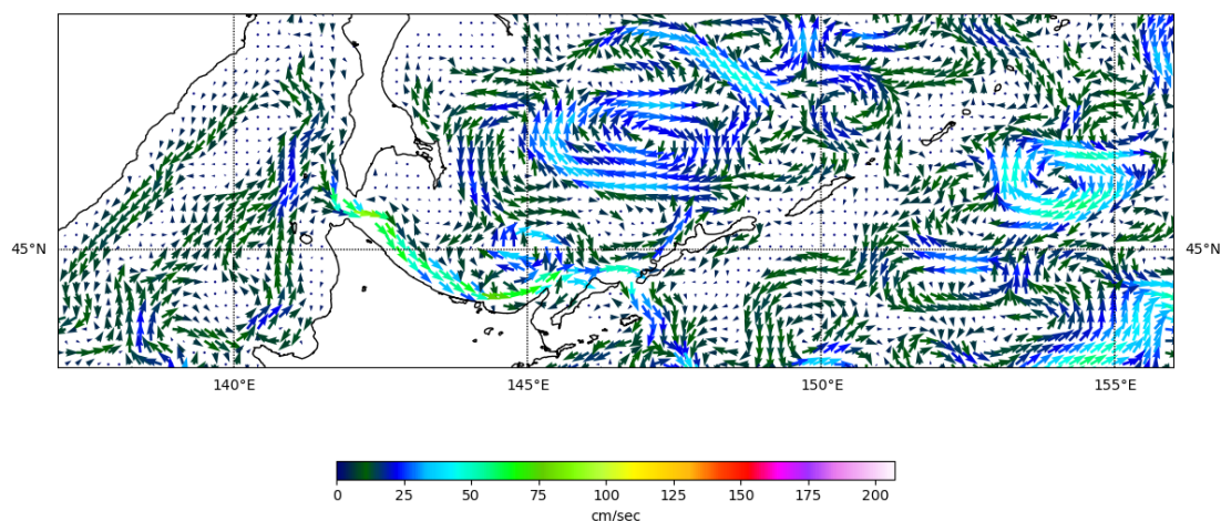
Рис. 3-7 Поверхностные течения, южная часть Охотского моря, 5 сентября 2022 г.
