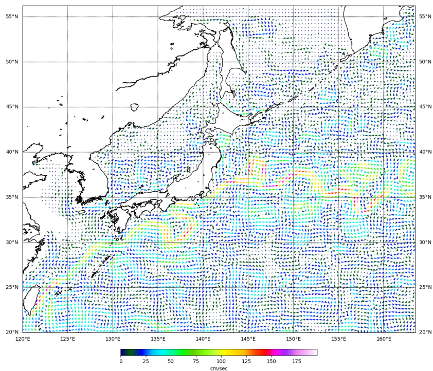
Рис. 3-5 Поверхностные течения западной части Тихого океана, 15 сентября 2022 г.
