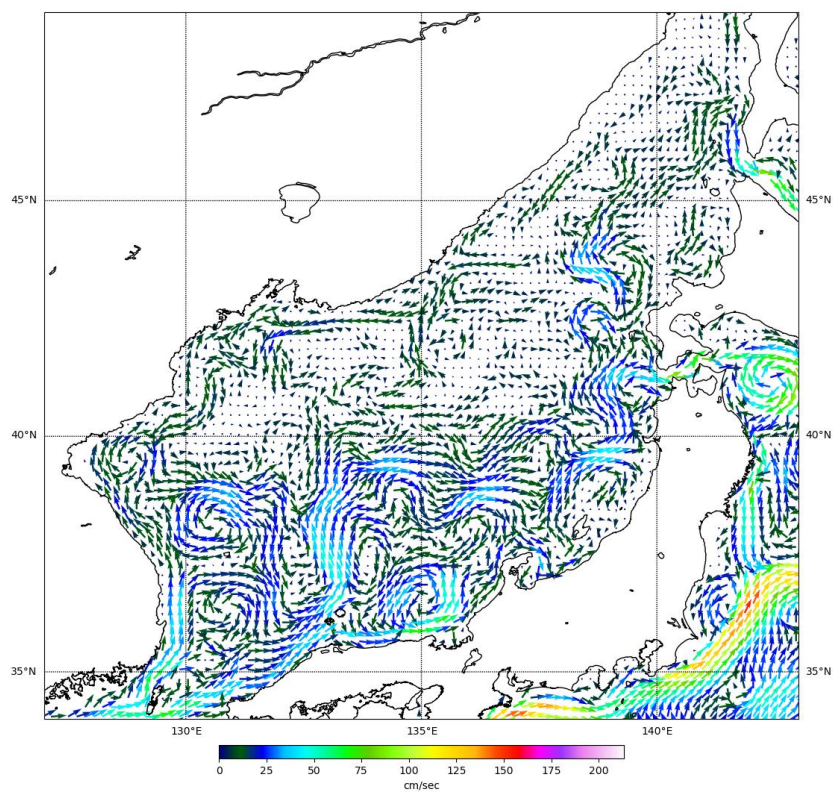
Рис. 3-3 Поверхностные течения Японского моря, 25 сентября 2022 г.
