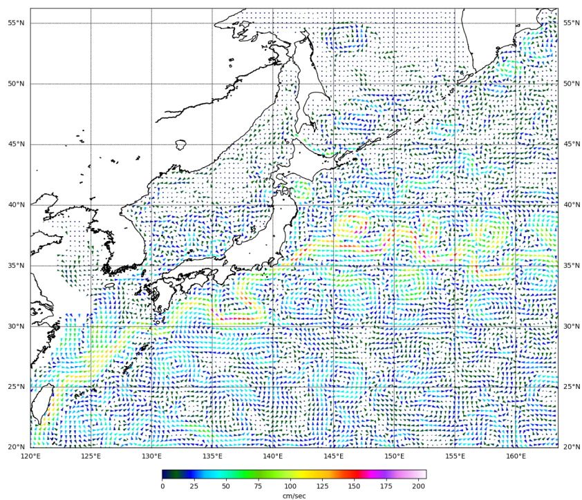
Рис. 3-4 Поверхностные течения западной части Тихого океана, 5 сентября 2022 г.
