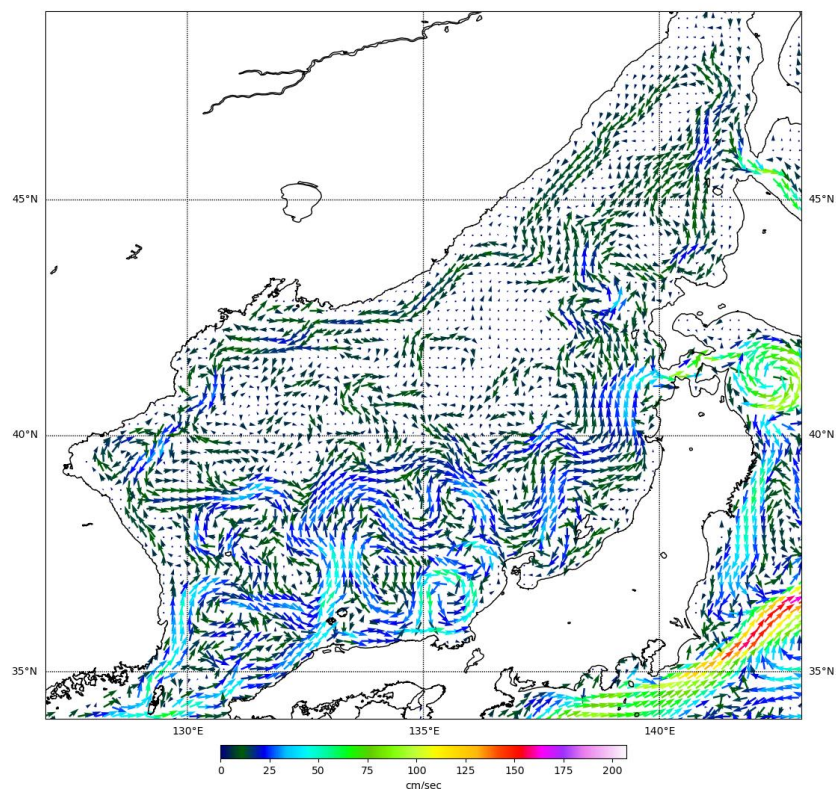
Рис. 3-1 Поверхностные течения Японского моря, 05 сентября 2022 г.
