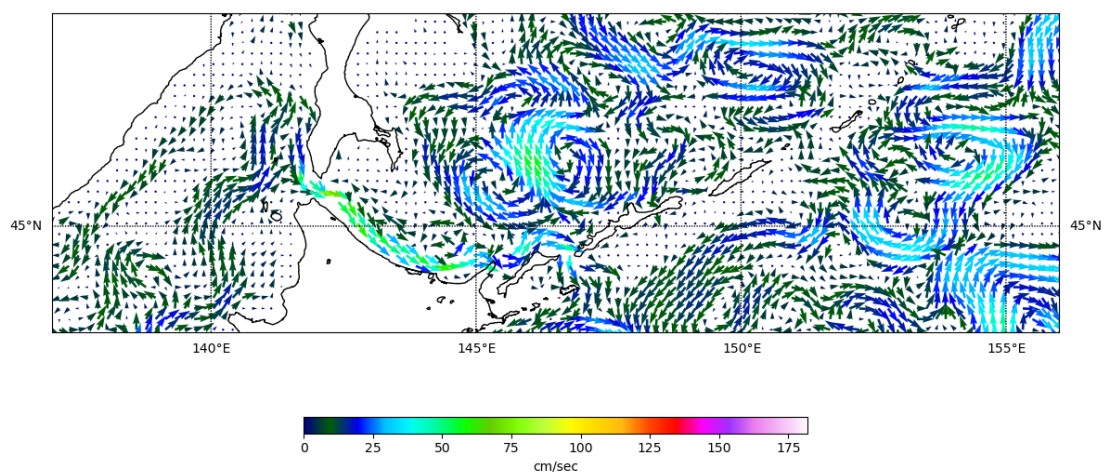
Рис. 3-8 Поверхностные течения, южная часть Охотского моря, 15 августа 2022 г.
