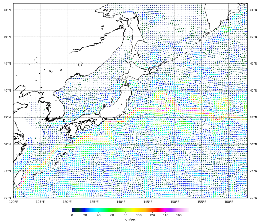
Рис. 3-5 Поверхностные течения западной части Тихого океана, 15 августа 2022 г.
