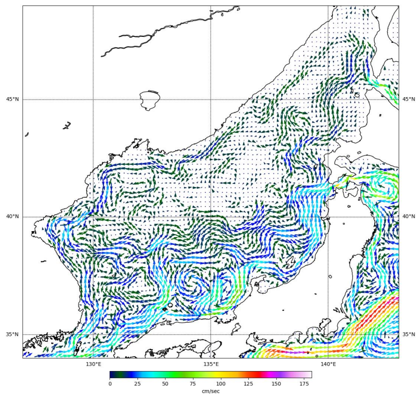
Рис. 3-2 Поверхностные течения Японского моря, 15 августа 2022 г.
