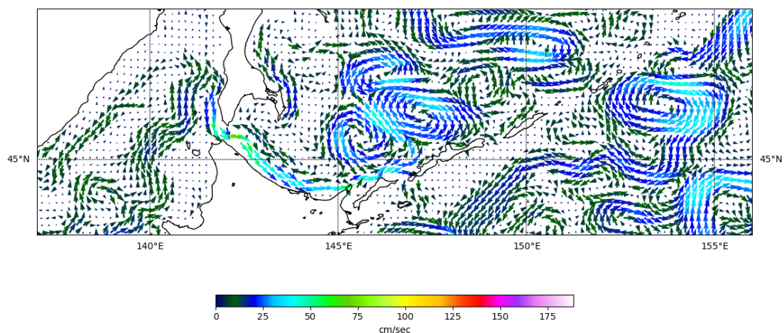
Рис. 3-7 Поверхностные течения, южная часть Охотского моря, 5 августа 2022 г.
