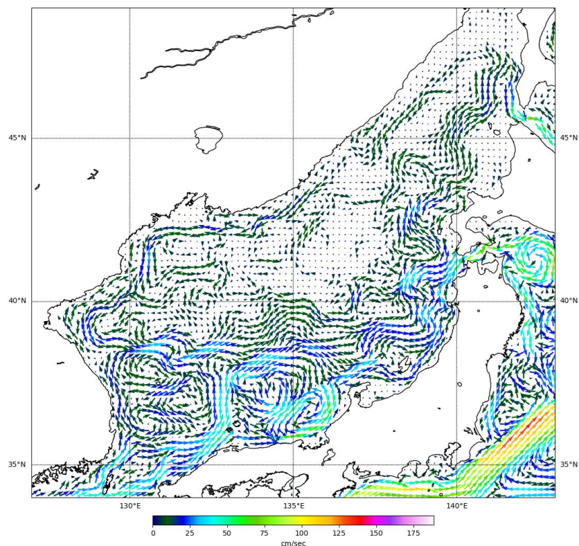
Рис. 3-1 Поверхностные течения Японского моря, 05 августа 2022 г.
