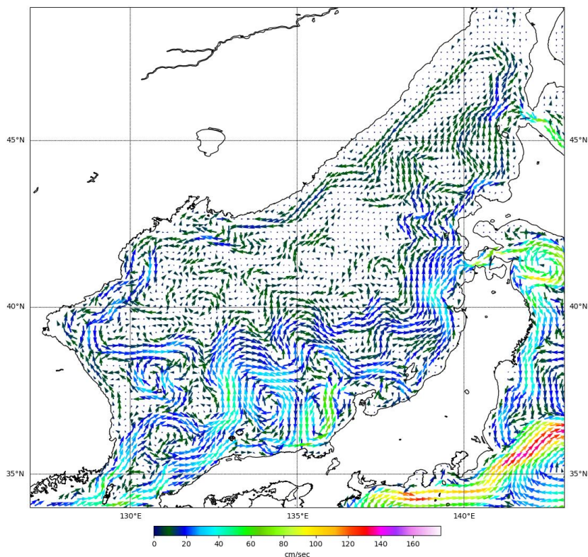
Рис. 3-3 Поверхностные течения Японского моря, 25 августа 2022 г.
