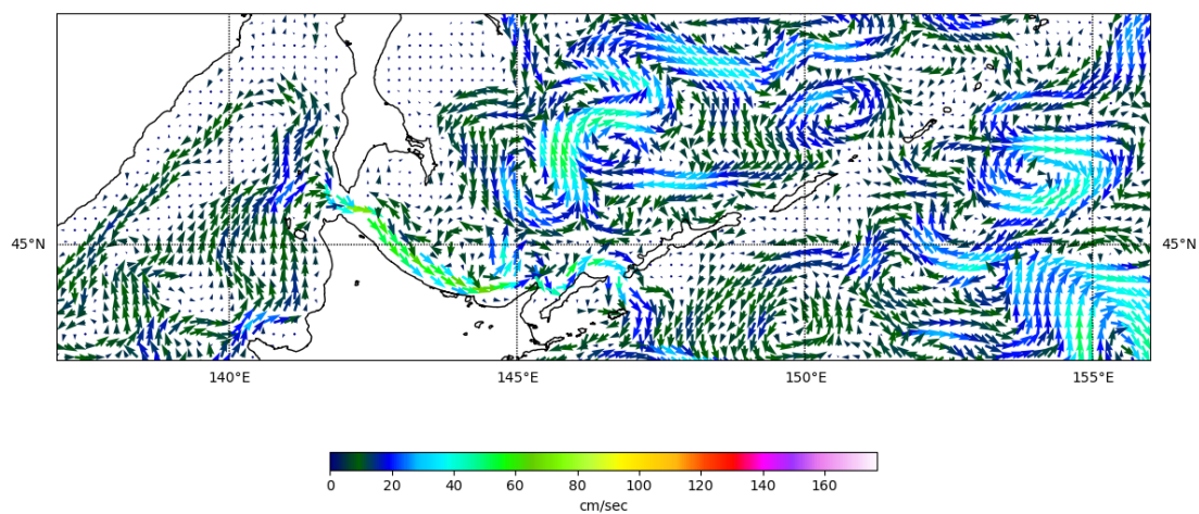
Рис. 3-9 Поверхностные течения, южная часть Охотского моря, 25 августа 2022 г.
