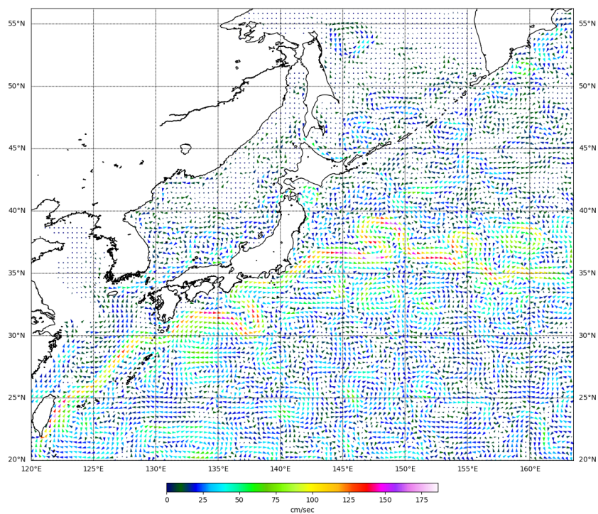
Рис. 3-4 Поверхностные течения западной части Тихого океана, 5 августа 2022 г.
