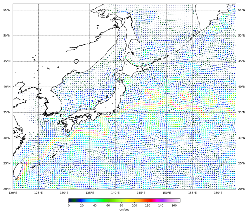
Рис. 3-6 Поверхностные течения западной части Тихого океана, 25 августа 2022 г.
