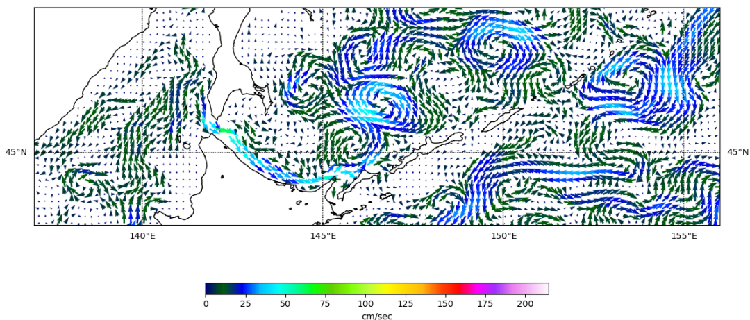
Рис. 3-7 Поверхностные течения, южная часть Охотского моря, 5 июля 2022 г.
