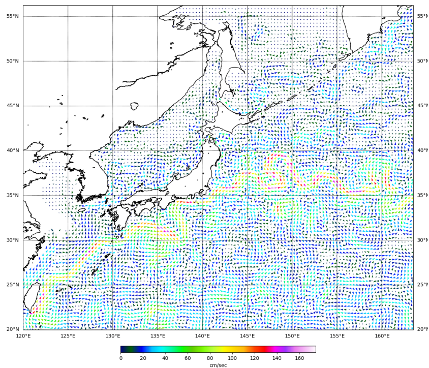
Рис. 3-5 Поверхностные течения западной части Тихого океана, 15 июля 2022 г.
