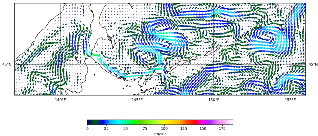
Рис. 3-9 Поверхностные течения, южная часть Охотского моря, 25 июля 2022 г.
