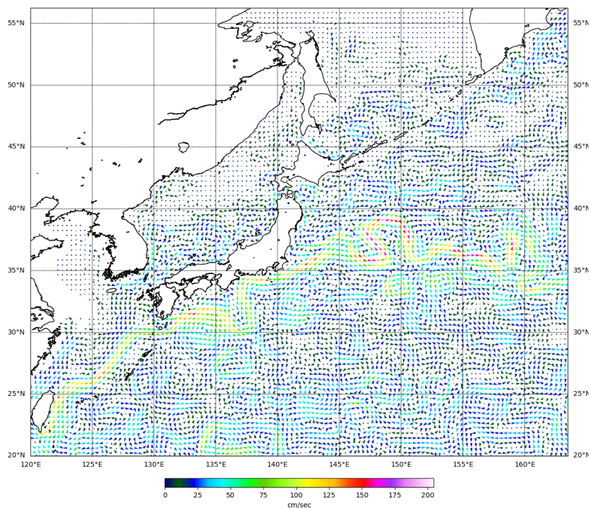
Рис. 3-4 Поверхностные течения западной части Тихого океана, 5 июля 2022 г.
