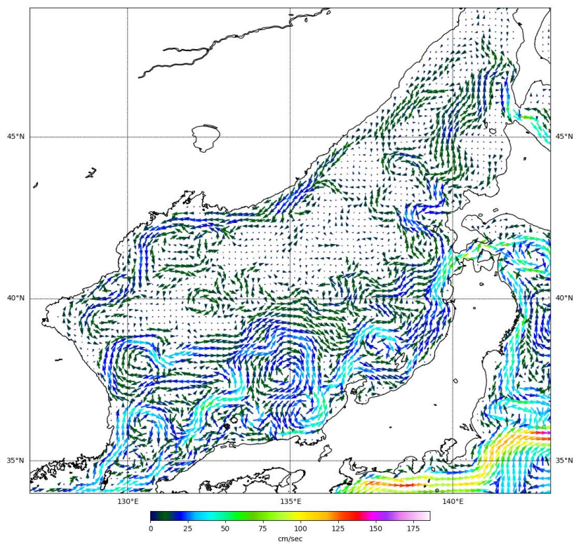
Рис. 3-2 Поверхностные течения Японского моря, 15 июля 2022 г.
