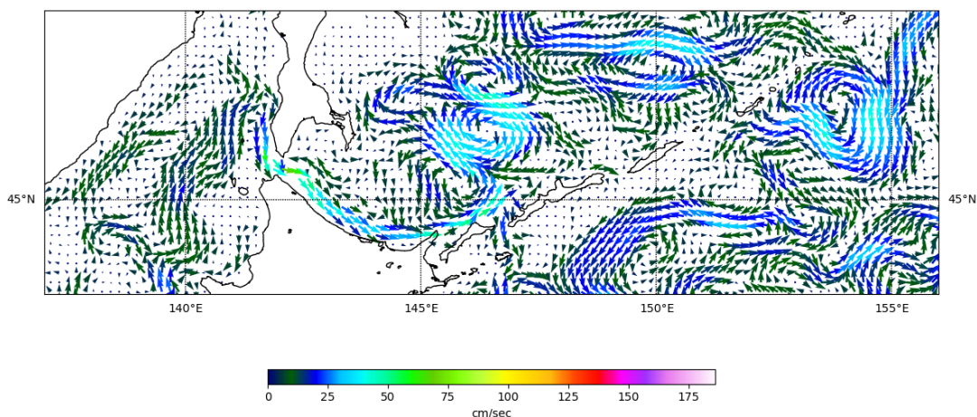
Рис. 3-8 Поверхностные течения, южная часть Охотского моря, 15 июля 2022 г.
