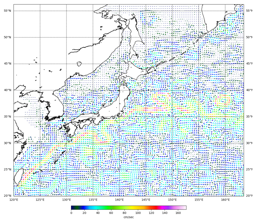
Рис. 3-6 Поверхностные течения западной части Тихого океана, 25 июля 2022 г.
