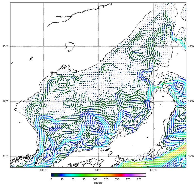
Рис. 3-1 Поверхностные течения Японского моря, 05 июля 2022 г.
