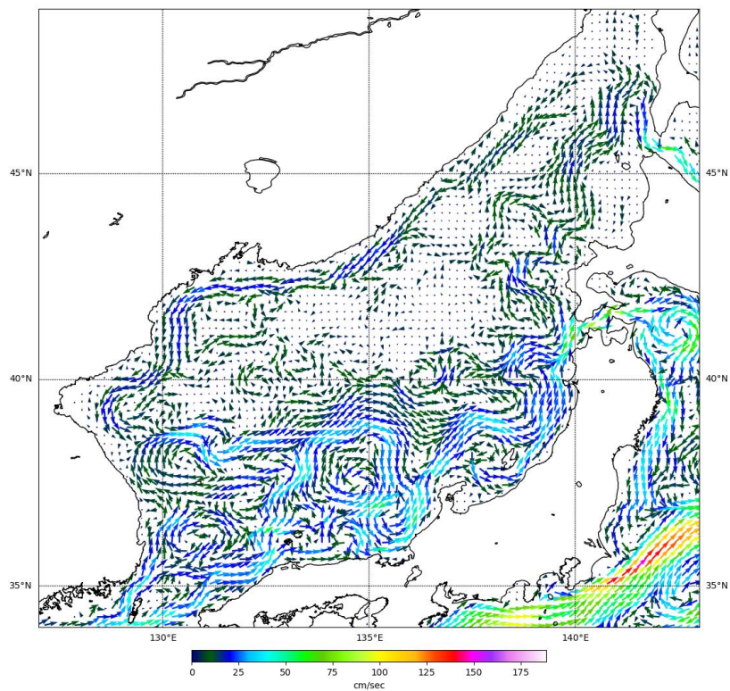
Рис. 3-3 Поверхностные течения Японского моря, 25 июля 2022 г.
