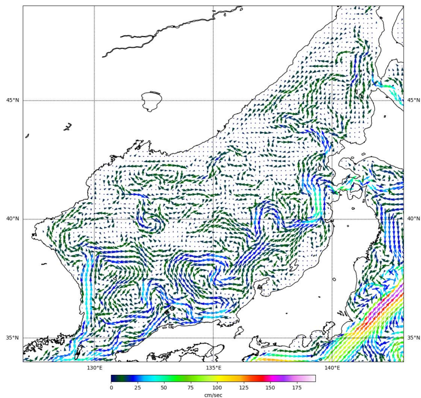
Рис. 3-2 Поверхностные течения Японского моря, 15 мая 2022 г.
