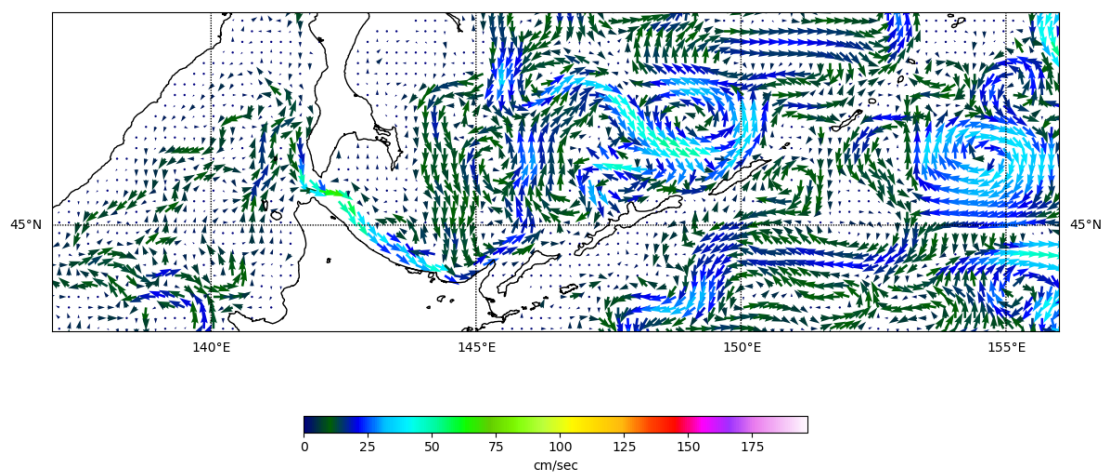
Рис. 3-9 Поверхностные течения, южная часть Охотского моря, 25 мая 2022 г.
