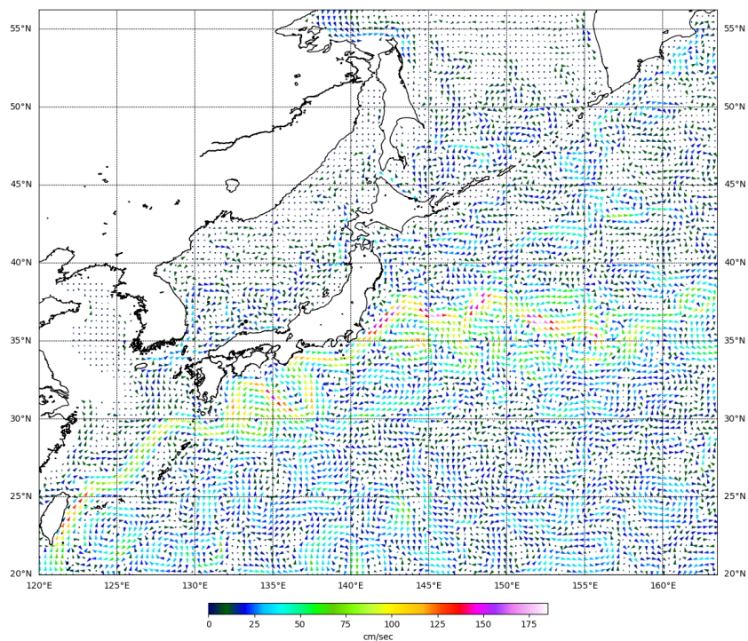
Рис. 3-5 Поверхностные течения западной части Тихого океана, 15 мая 2022 г.
