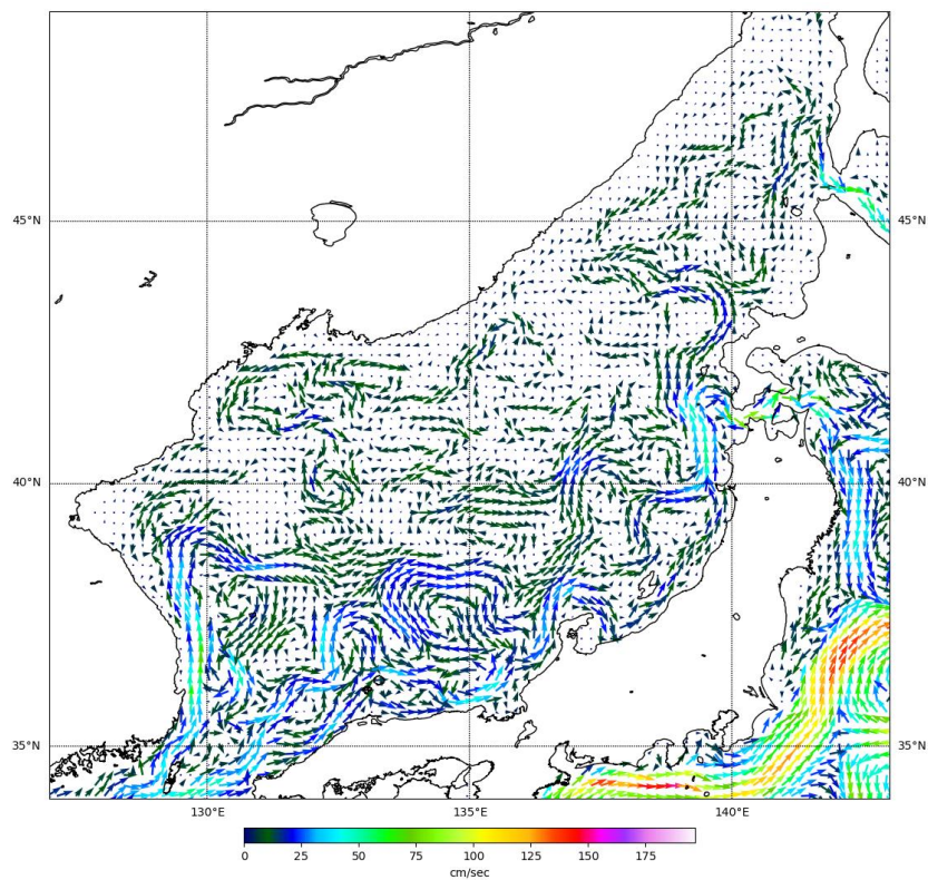
Рис. 3-3 Поверхностные течения Японского моря, 25 мая 2022 г.
