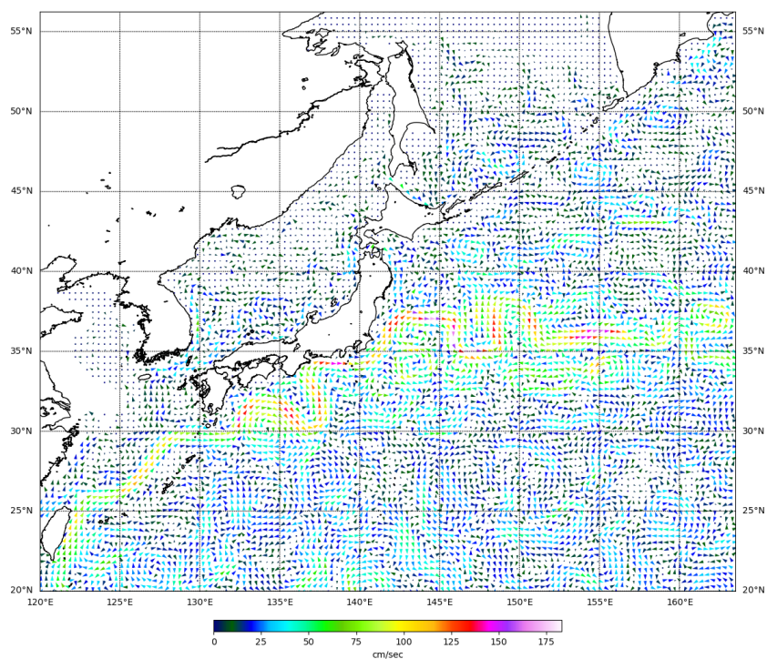
Рис. 3-6 Поверхностные течения западной части Тихого океана, 25 мая 2022 г.
