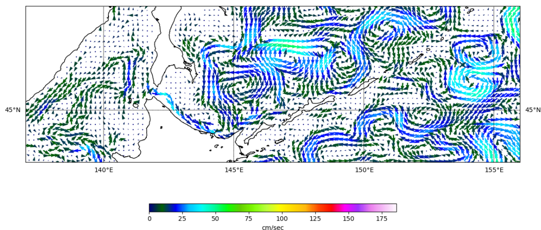
Рис. 3-7 Поверхностные течения, южная часть Охотского моря, 5 мая 2022 г.
