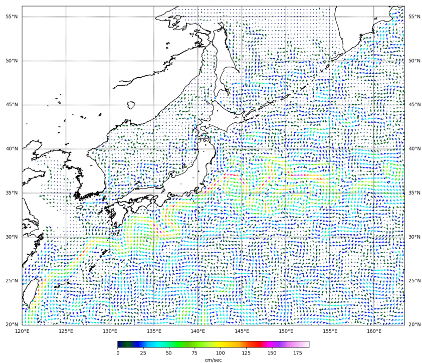
Рис. 3-4 Поверхностные течения западной части Тихого океана, 5 мая 2022 г.
