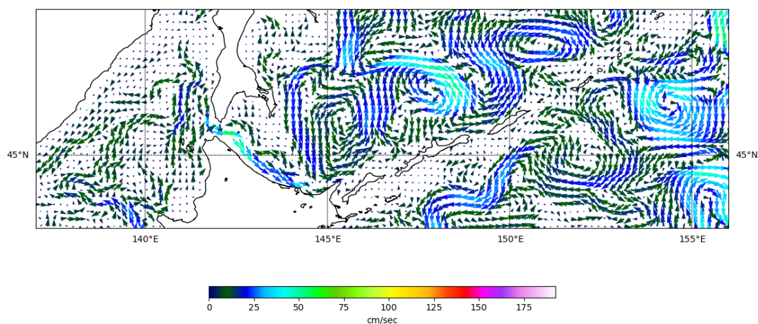
Рис. 3-8 Поверхностные течения, южная часть Охотского моря, 15 мая 2022 г.
