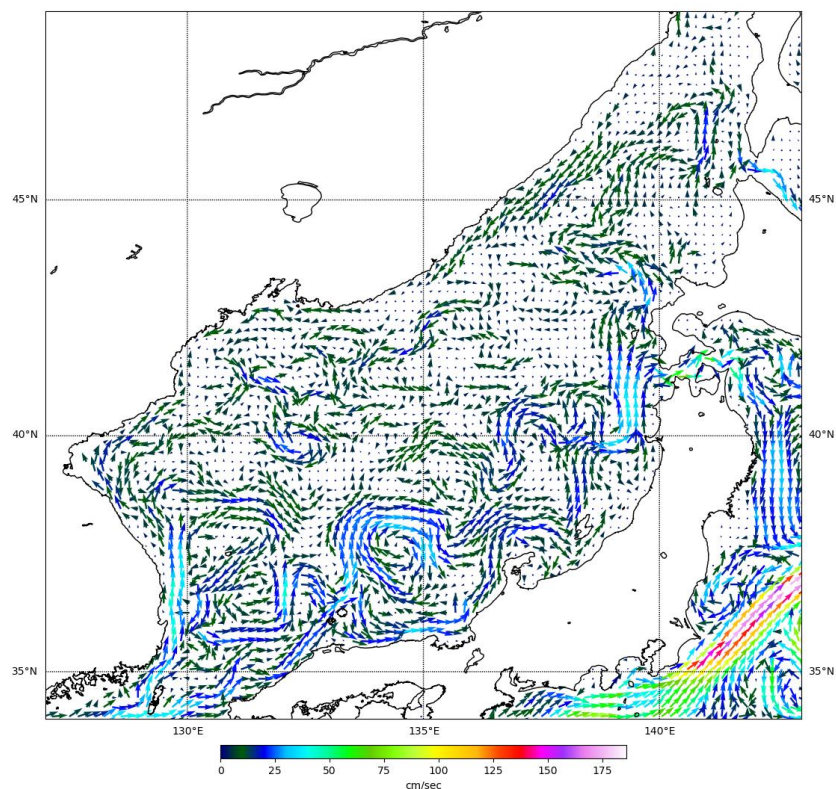
Рис. 3-1 Поверхностные течения Японского моря, 05 мая 2022 г.
