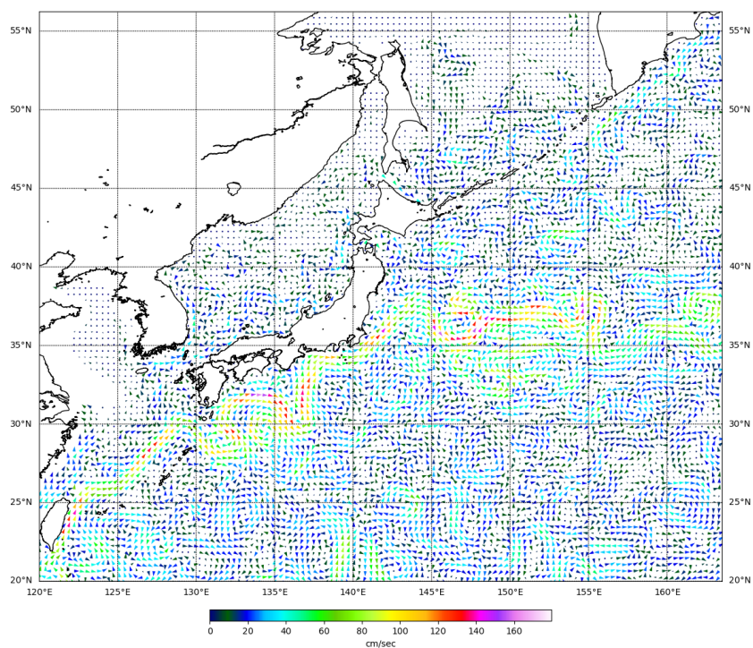
Рис. 3-6 Поверхностные течения западной части Тихого океана, 25 апреля 2022 г.
