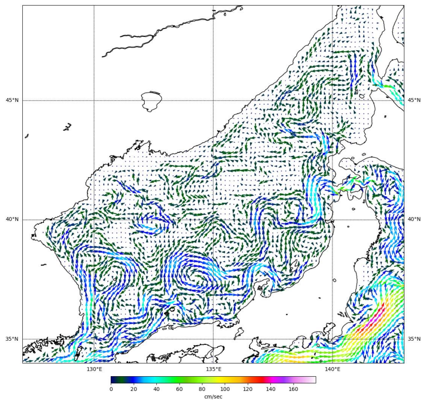
Рис. 3-3 Поверхностные течения Японского моря, 25 апреля 2022 г.
