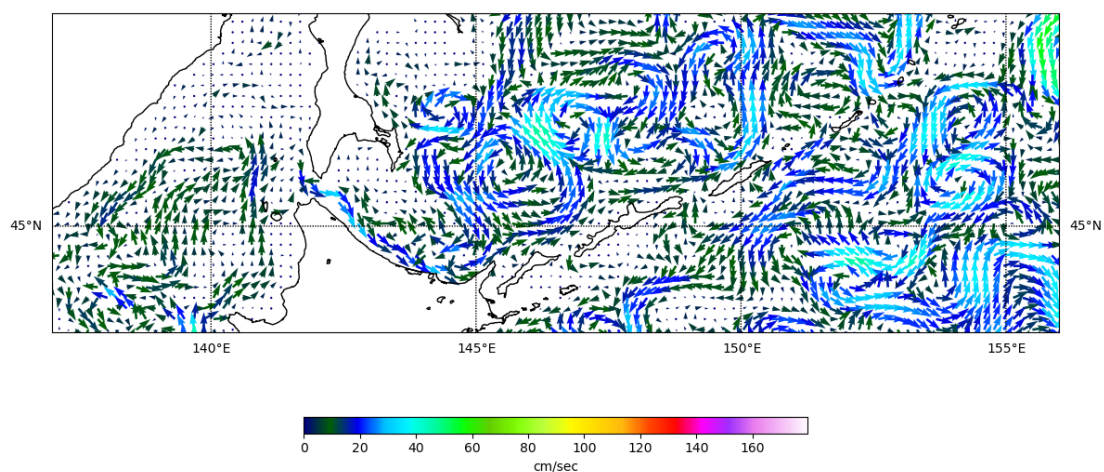
Рис. 3-8 Поверхностные течения, южная часть Охотского моря, 15 апреля 2022 г.
