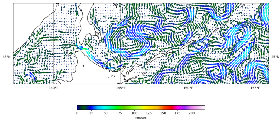
Рис. 3-7 Поверхностные течения, южная часть Охотского моря, 5 апреля 2022 г.
