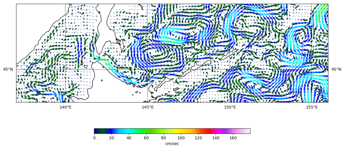
Рис. 3-9 Поверхностные течения, южная часть Охотского моря, 25 апреля 2022 г.
