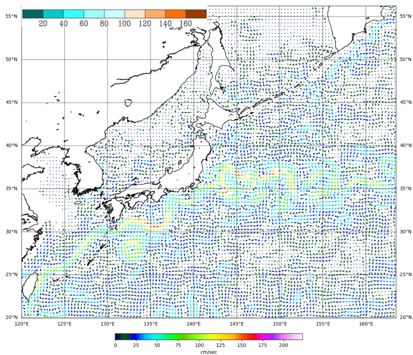
Рис. 3-4 Поверхностные течения западной части Тихого океана, 5 апреля 2022 г.
