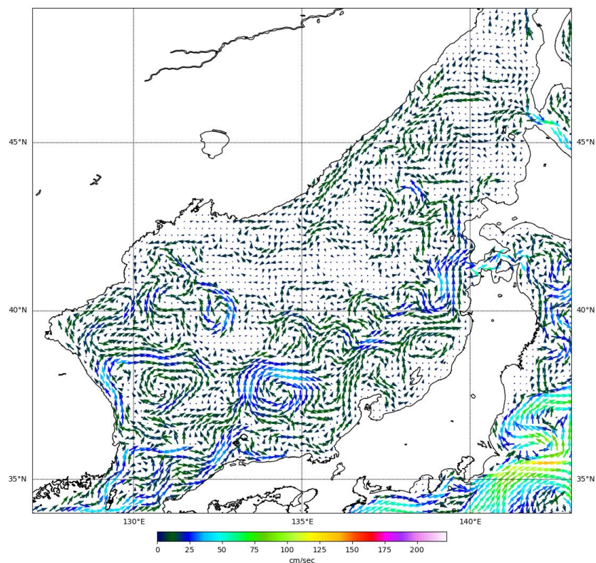
Рис. 3-1 Поверхностные течения Японского моря, 05 апреля 2022 г.
