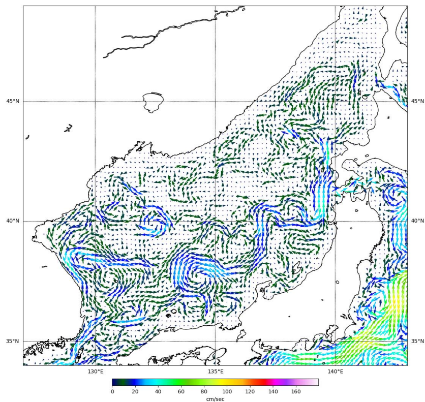
Рис. 3-2 Поверхностные течения Японского моря, 15 апреля 2022 г.
