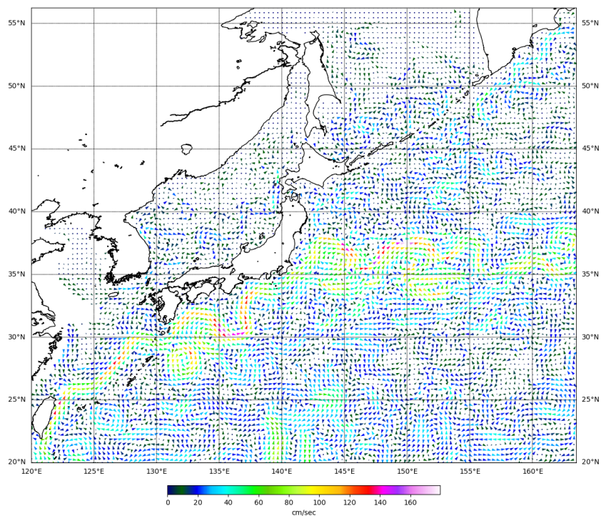
Рис. 3-5 Поверхностные течения западной части Тихого океана, 15 апреля 2022 г.
