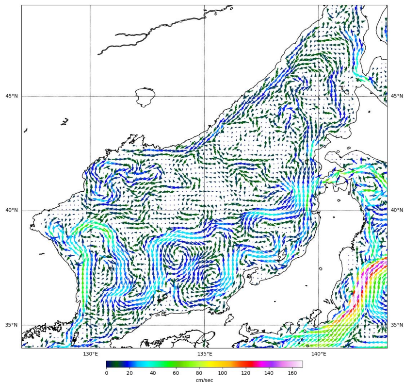
Рис. 3- Поверхностные течения Японского моря, 25 декабря 2022 г.
