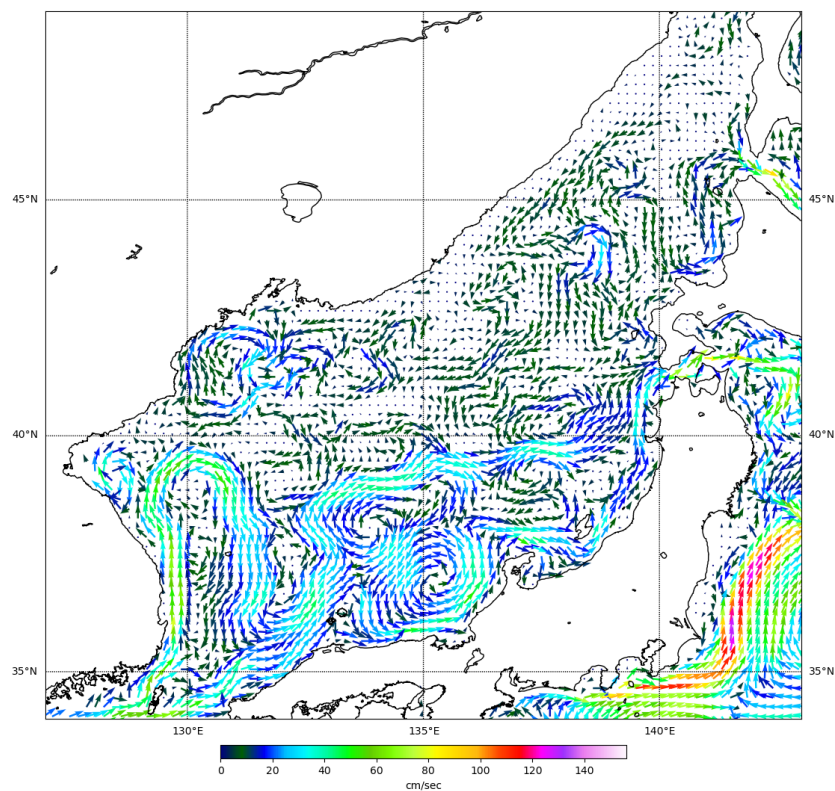
Рис. 3- Поверхностные течения Японского моря, 15 декабря 2022 г.
