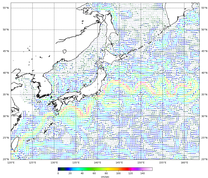
Рис. 3- Поверхностные течения западной части Тихого океана, 15 декабря 2022 г.
