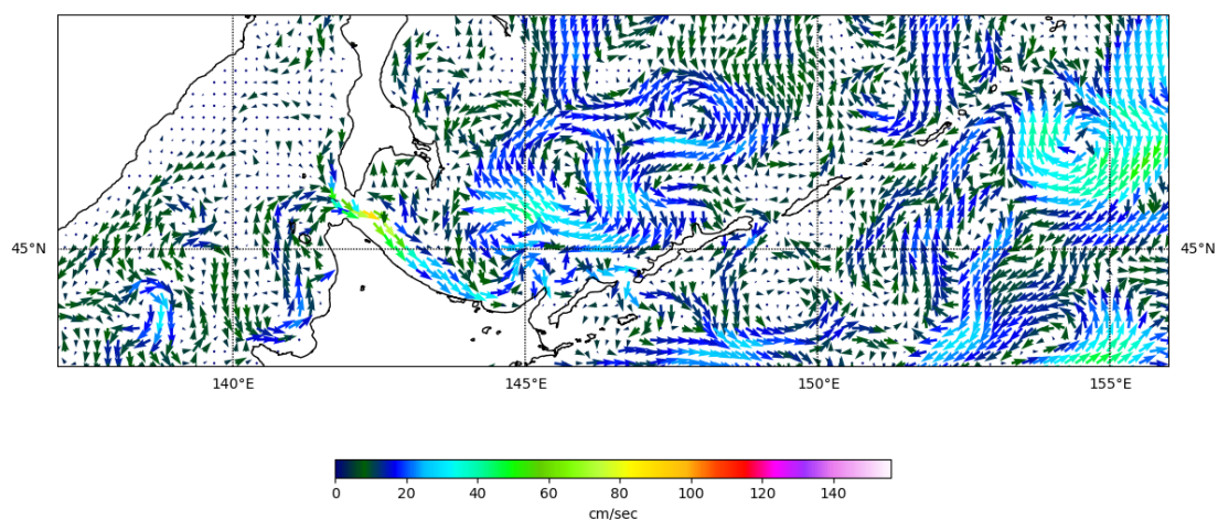
Рис. 3- Поверхностные течения, южная часть Охотского моря, 15 декабря 2022 г.
