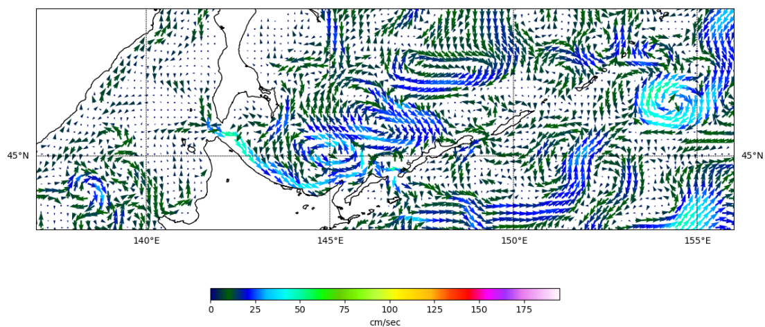
Рис. 3- Поверхностные течения, южная часть Охотского моря, 5 декабря 2022 г.
