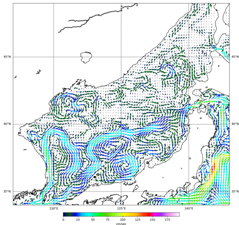
Рис. 3- Поверхностные течения Японского моря, 05 декабря 2022 г.
