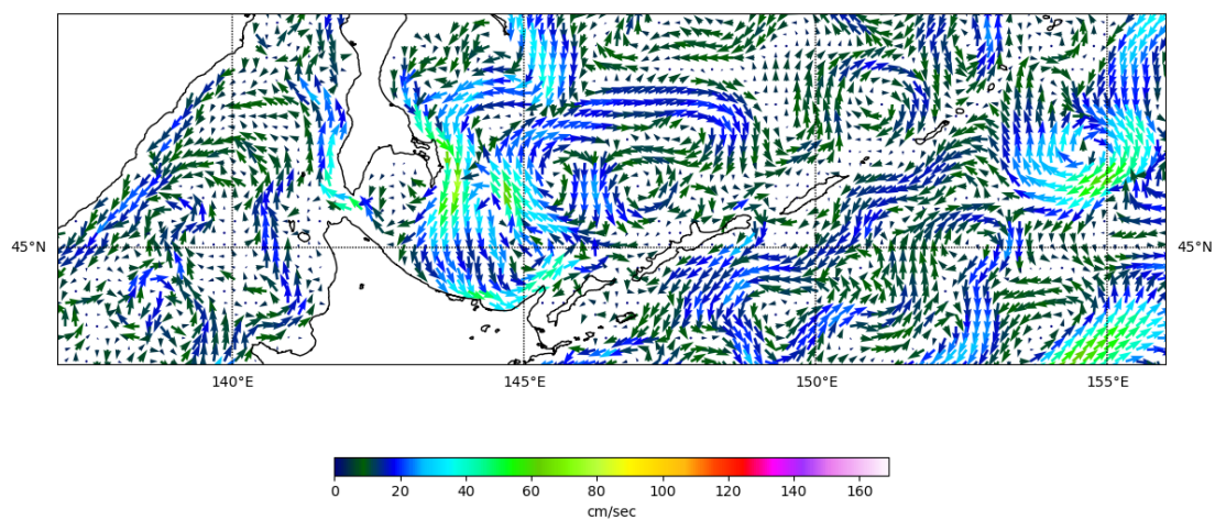
Рис. 3- Поверхностные течения, южная часть Охотского моря, 25 октября 2022 г.
