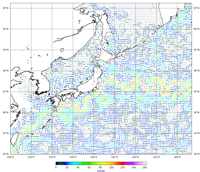
Рис. 3- Поверхностные течения западной части Тихого океана, 25 декабря 2022 г.
