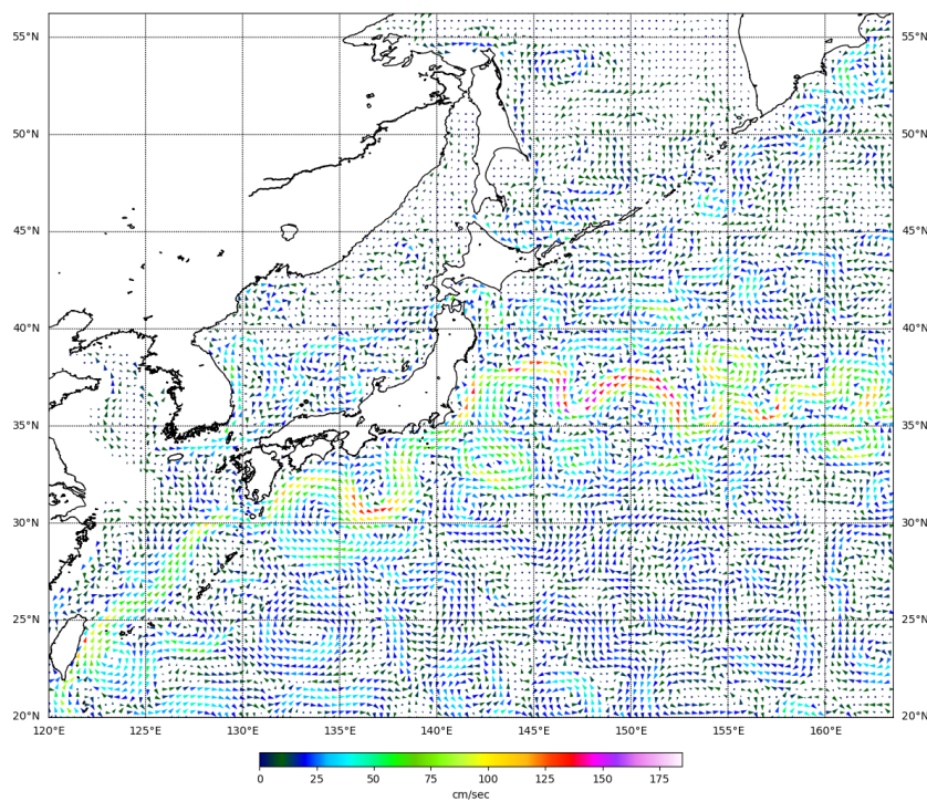
Рис. 3- Поверхностные течения западной части Тихого океана, 5 декабря 2022 г.
