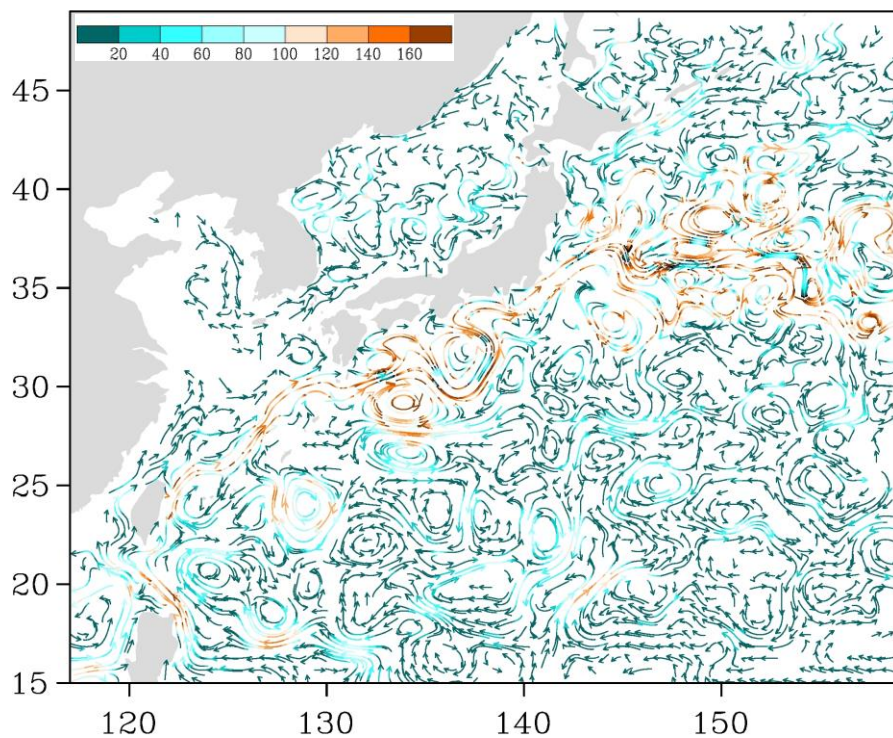
Рис. 3-5 Поверхностные течения западной части Тихого океана, 15 января 2022 г.
