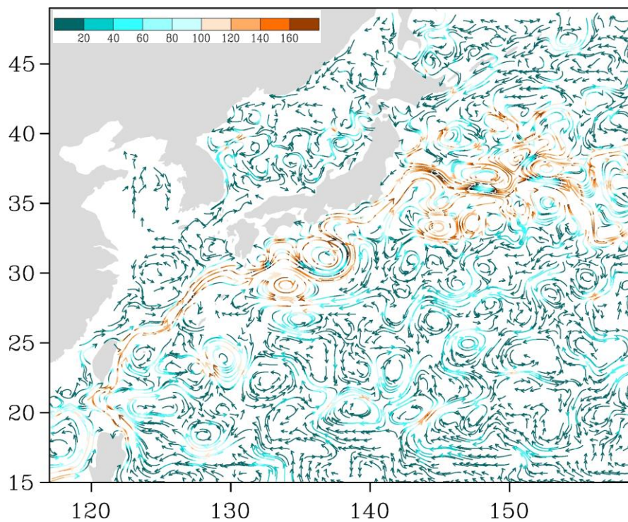
Рис. 3-4 Поверхностные течения западной части Тихого океана, 5 января 2022 г.
