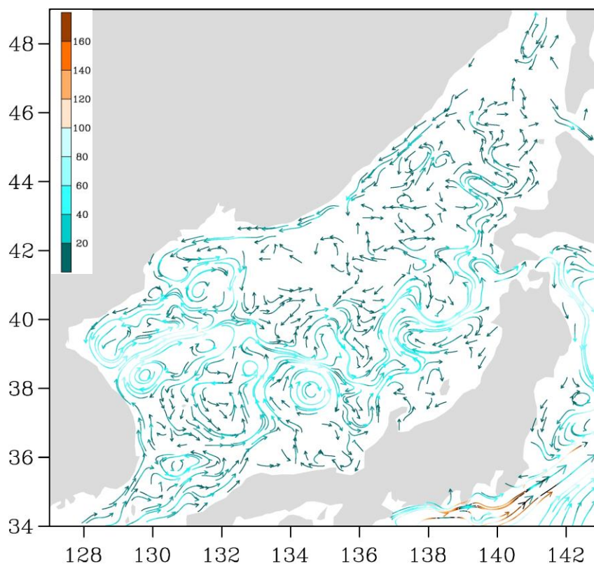
Рис. 3-3 Поверхностные течения Японского моря, 25 января 2022 г.
