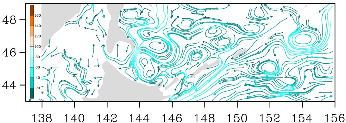
Рис. 3-7 Поверхностные течения, южная часть Охотского моря, 5 января 2022 г.
