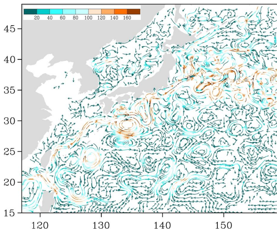
Рис. 3-6 Поверхностные течения западной части Тихого океана, 25 января 2022 г.
