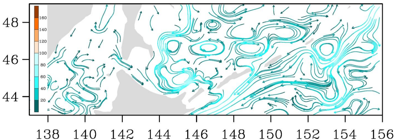
Рис. 3-9 Поверхностные течения, южная часть Охотского моря, 25 января 2022 г.
