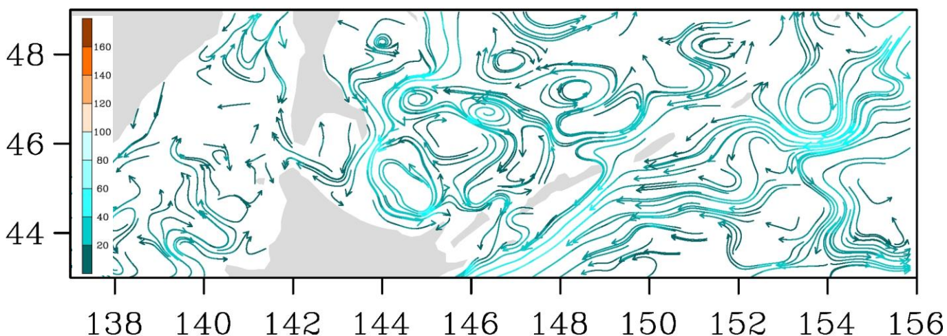
Рис. 3-8 Поверхностные течения, южная часть Охотского моря, 15 января 2022 г.
