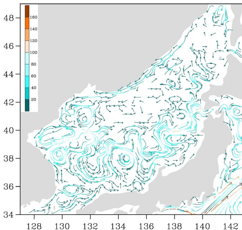
Рис. 3-2 Поверхностные течения Японского моря, 15 января 2022 г.
