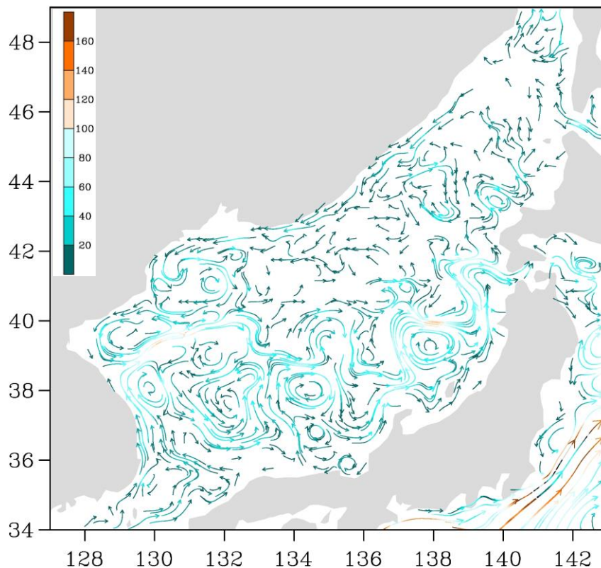
Рис. 3-1 Поверхностные течения Японского моря, 05 января 2022 г.
