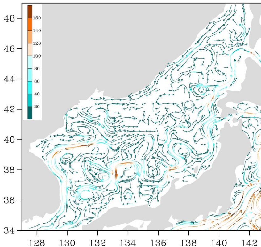
Рис. 3-1 Поверхностные течения Японского моря, 05 декабря 2021 г.
