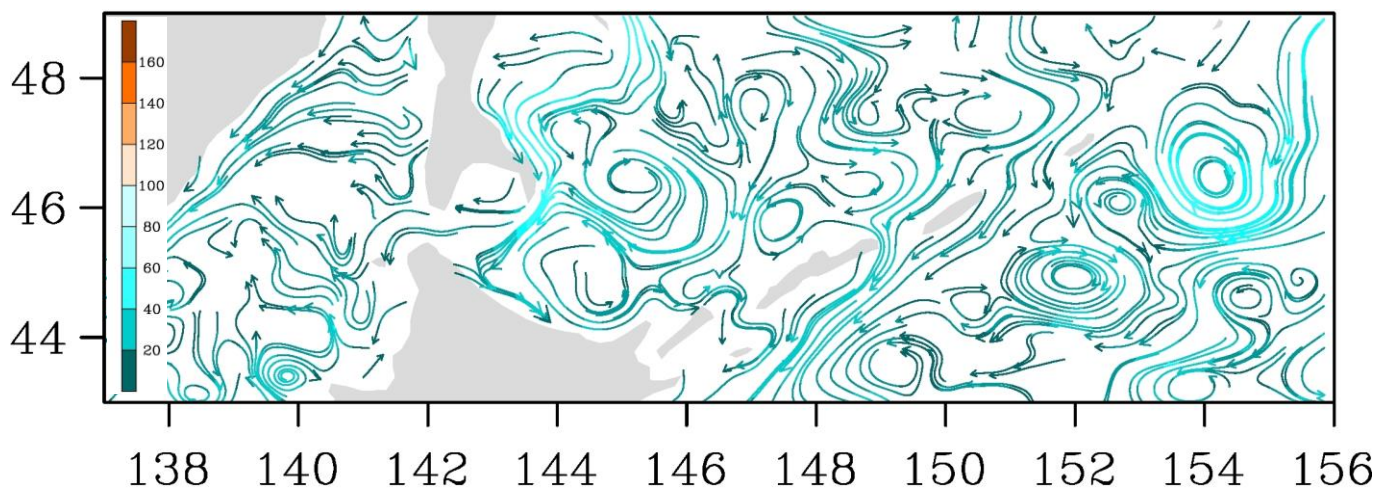
Рис. 3-9 Поверхностные течения, южная часть Охотского моря, 25 декабря 2021 г.
