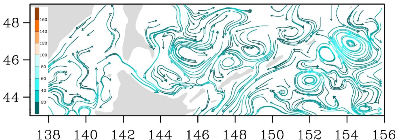
Рис. 3-8 Поверхностные течения, южная часть Охотского моря, 15 декабря 2021 г.
