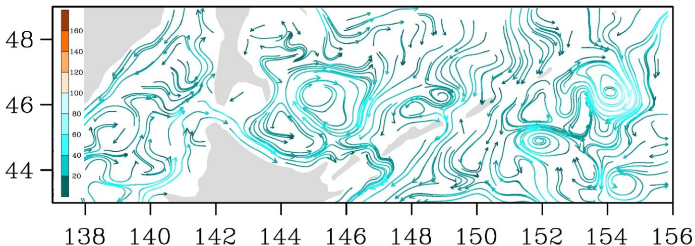
Рис. 3-7 Поверхностные течения, южная часть Охотского моря, 5 декабря 2021 г.
