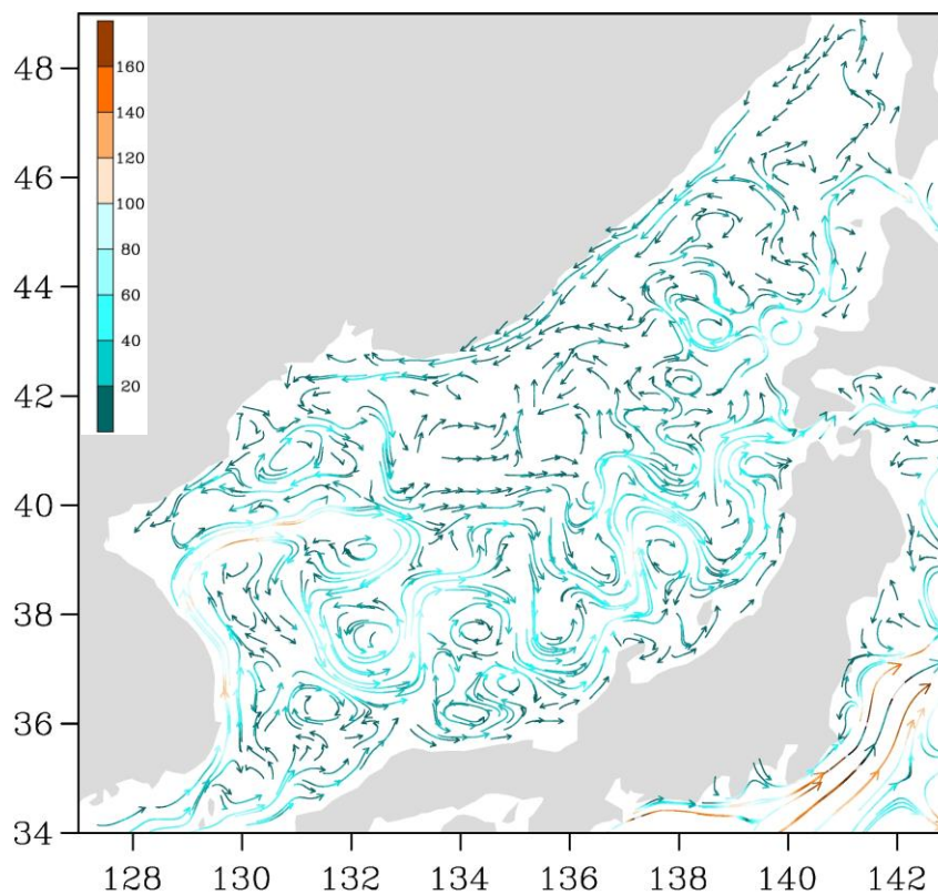
Рис. 3-2 Поверхностные течения Японского моря, 15 декабря 2021 г.
