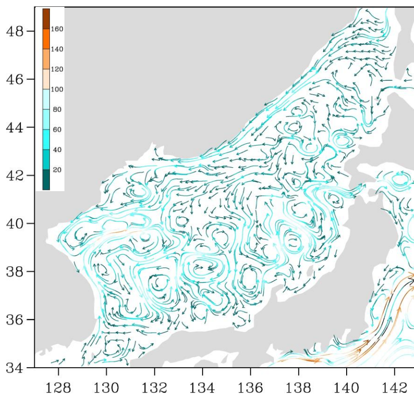
Рис. 3-3 Поверхностные течения Японского моря, 25 декабря 2021 г.
