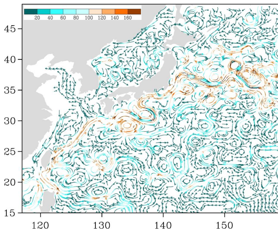
Рис. 3-6 Поверхностные течения западной части Тихого океана, 25 декабря 2021 г.
