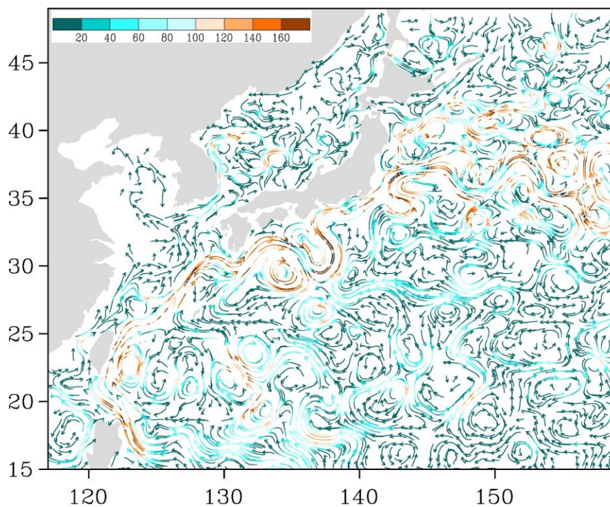
Рис. 3-4 Поверхностные течения западной части Тихого океана, 5 декабря 2021 г.
