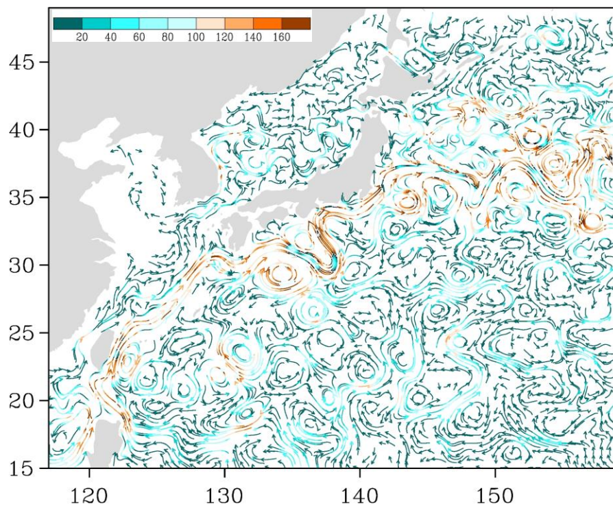
Рис. 3-5 Поверхностные течения западной части Тихого океана, 15 декабря 2021 г.
