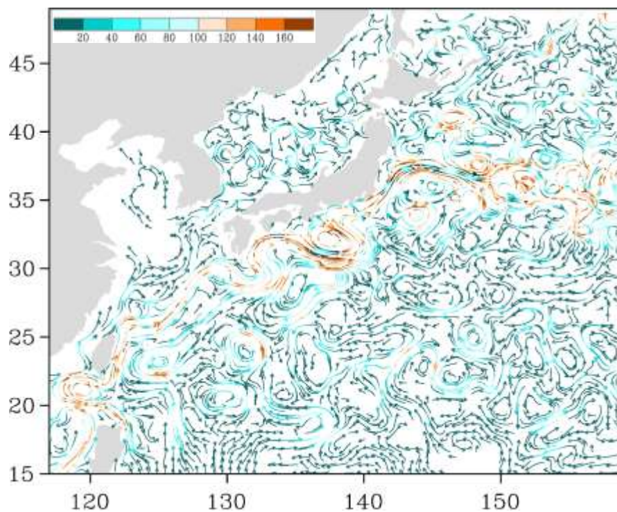
Рис. 3-4 Поверхностные течения западной части Тихого океана, 5 февраля 2021 г.
