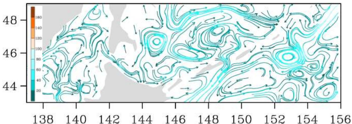
Рис. 3-8 Поверхностные течения, пролив Лаперуза, 15 февраля 2021 г.
