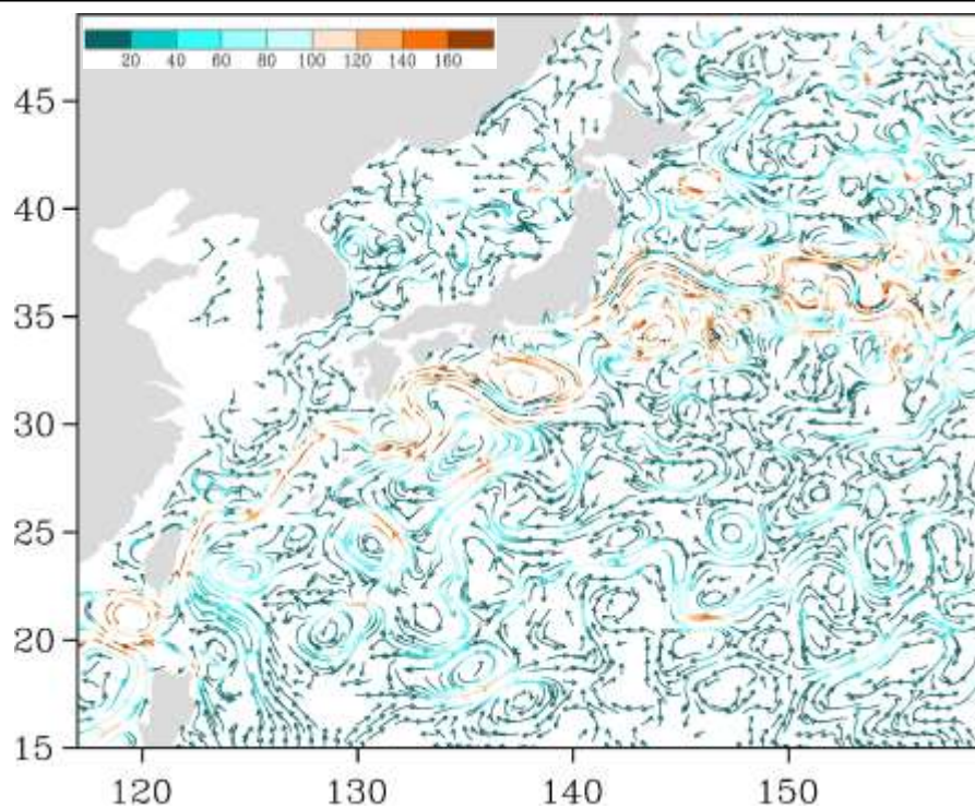
Рис. 3-5 Поверхностные течения западной части Тихого океана, 15 февраля 2021 г.
