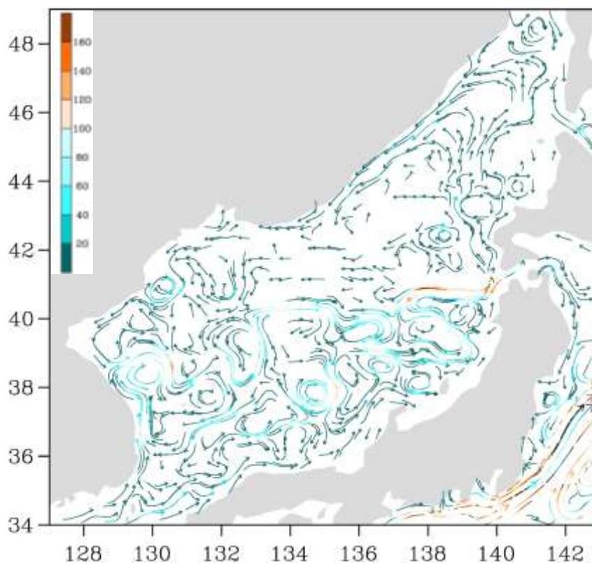
Рис. 3-2 Поверхностные течения Японского моря, 15 февраля 2021 г.
