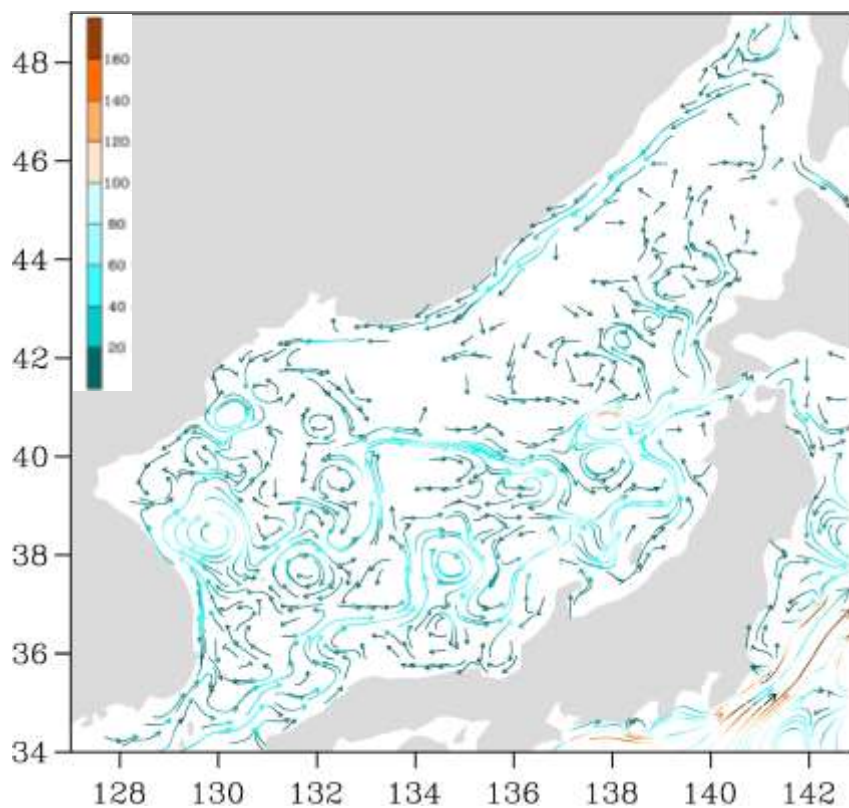
Рис. 3-3 Поверхностные течения Японского моря, 25 февраля 2021 г.
