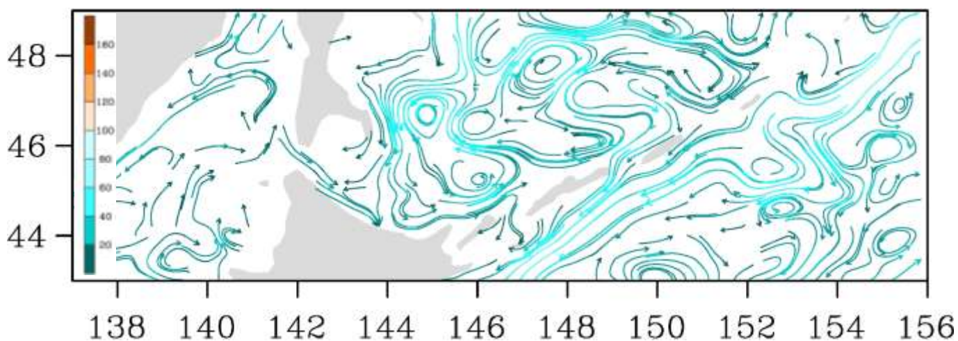
Рис. 3-9 Поверхностные течения, пролив Лаперуза, 25 февраля 2021 г.
