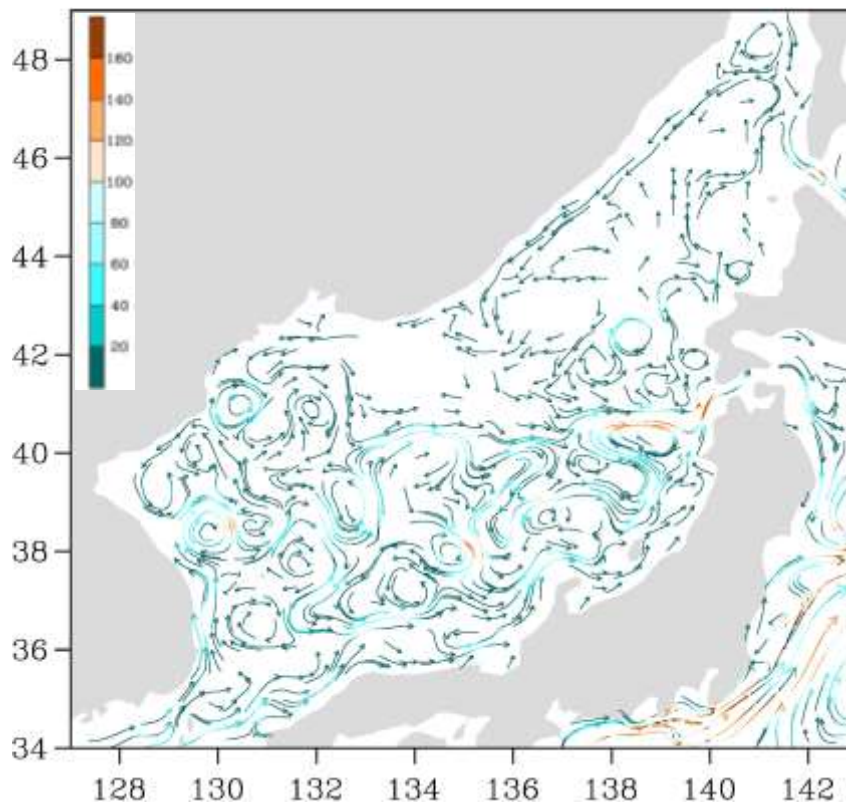
Рис. 3-1 Поверхностные течения Японского моря, 05 февраля 2021 г.
