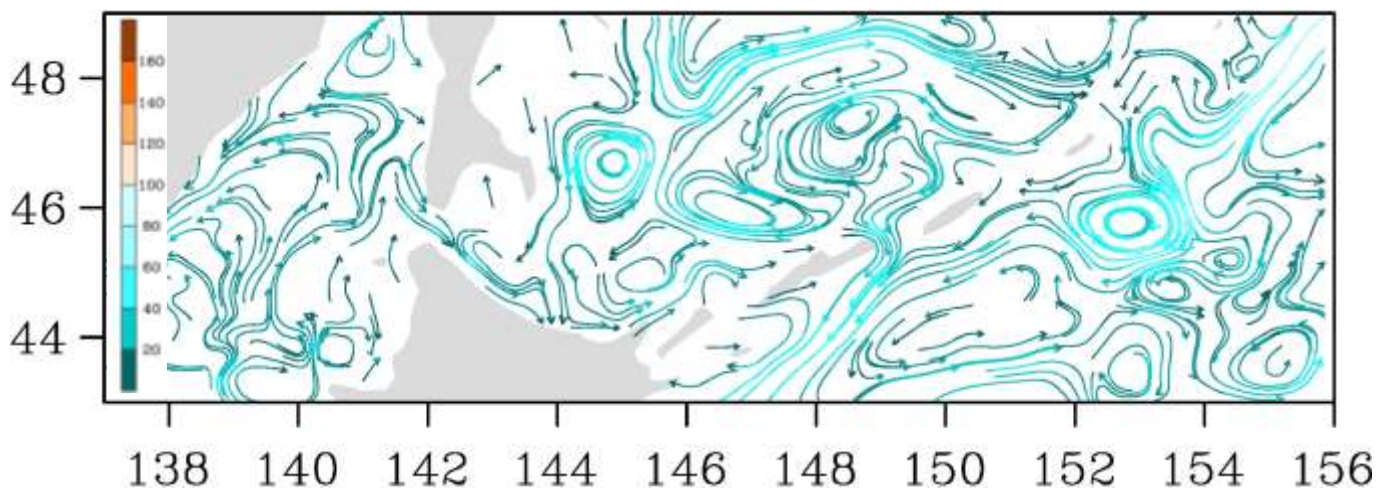
Рис. 3-7 Поверхностные течения, пролив Лаперуза, 5 февраля 2021 г.
