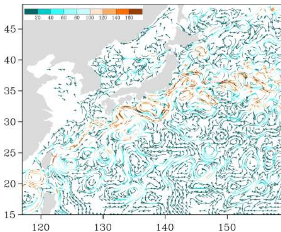
Рис. 3-6 Поверхностные течения западной части Тихого океана, 25 февраля 2021 г.
