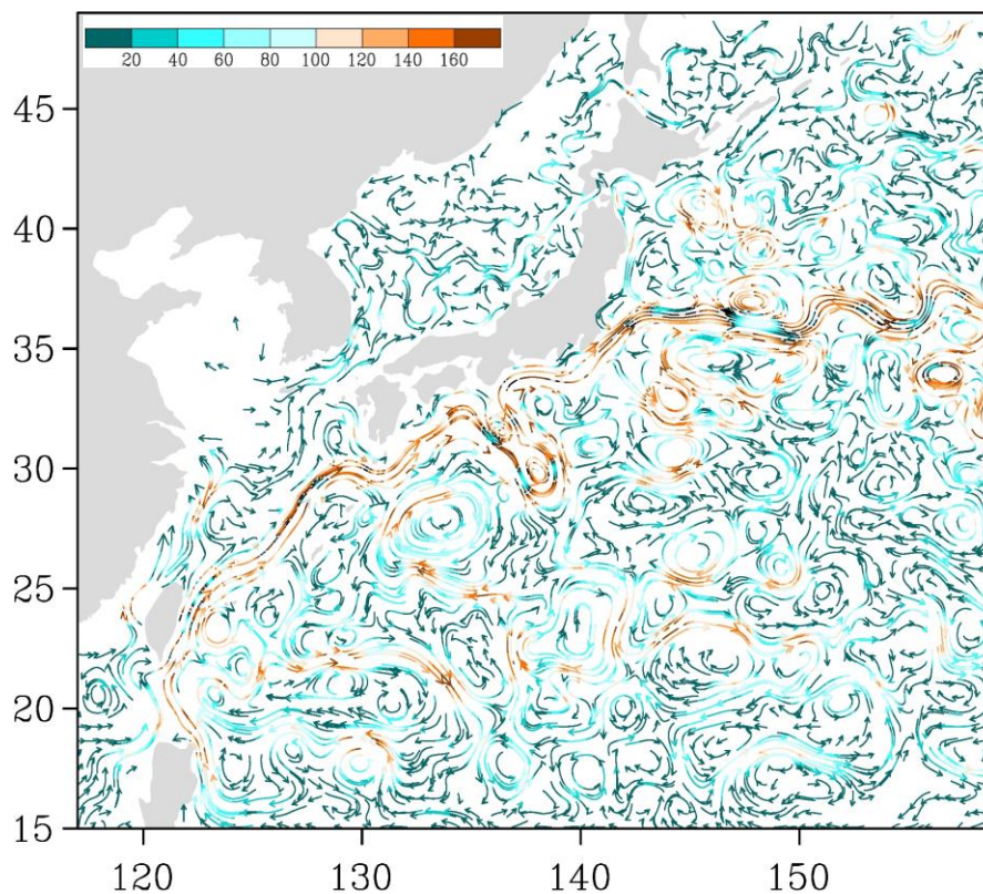
Рис. 3-4 Поверхностные течения западной части Тихого океана, 5 августа 2020 г.
