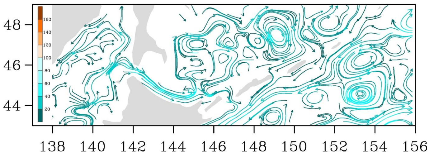
Рис. 3-9 Поверхностные течения, пролив Лаперуза, 25 августа 2020 г.
