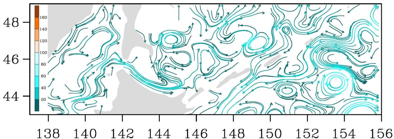
Рис. 3-7 Поверхностные течения, пролив Лаперуза, 5 августа 2020 г.
