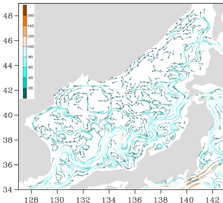
Рис. 3-3 Поверхностные течения Японского моря, 25 августа 2020 г.
