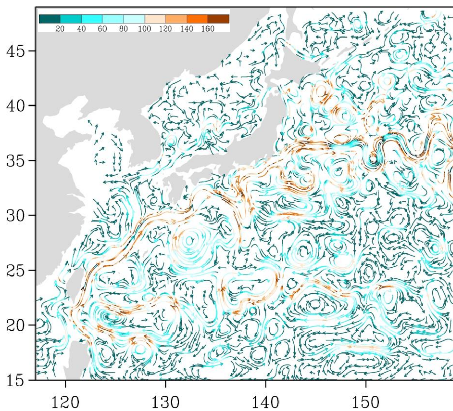
Рис. 3-6 Поверхностные течения западной части Тихого океана, 25 августа 2020 г.
