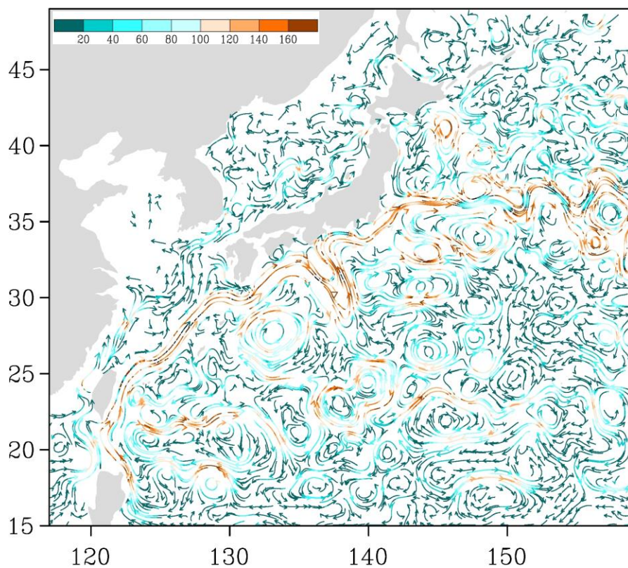
Рис. 3-5 Поверхностные течения западной части Тихого океана, 15 августа 2020 г.
