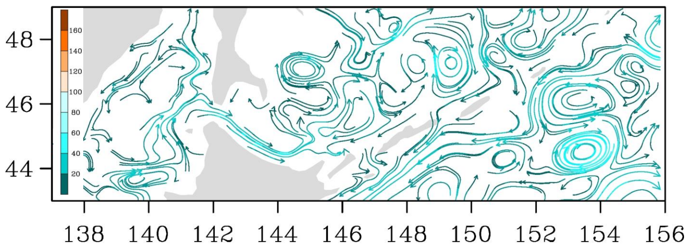
Рис. 3-8 Поверхностные течения, пролив Лаперуза, 15 августа 2020 г.
