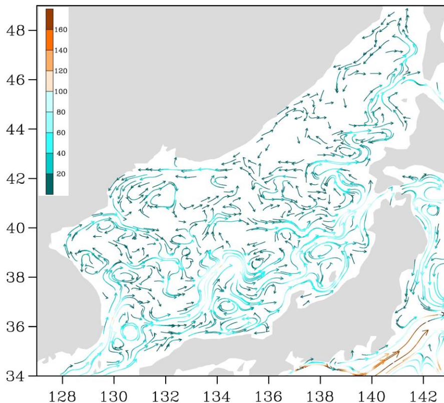
Рис. 3-2 Поверхностные течения Японского моря, 15 августа 2020 г.
