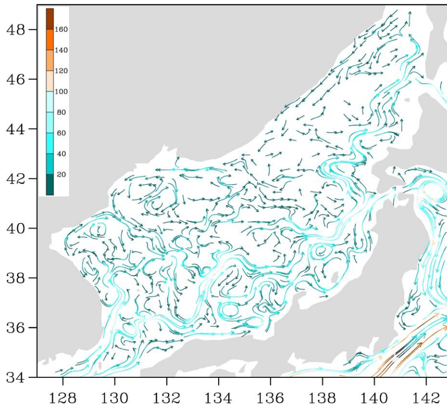
Рис. 3-1 Поверхностные течения Японского моря, 05 августа 2020 г.
