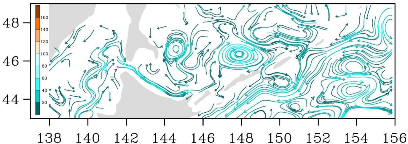
Рис. 3-8 Поверхностные течения, пролив Лаперуза, 15 июня 2020 г.
