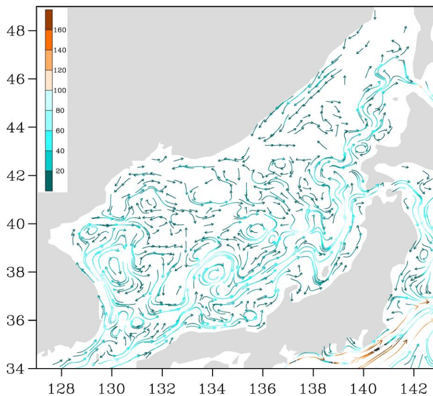
Рис. 3-2 Поверхностные течения Японского моря, 15 июня 2020 г.
