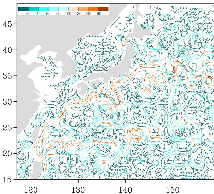
Рис. 3-6 Поверхностные течения западной части Тихого океана, 25 июня 2020 г.
