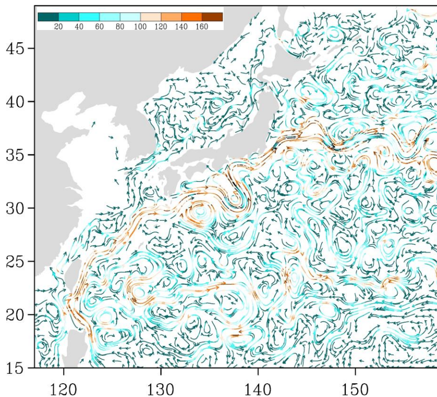
Рис. 3-4 Поверхностные течения западной части Тихого океана, 5 июня 2020 г.
