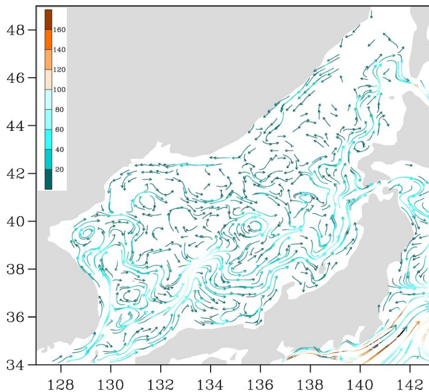
Рис. 3-1 Поверхностные течения Японского моря, 05 июня 2020 г.
