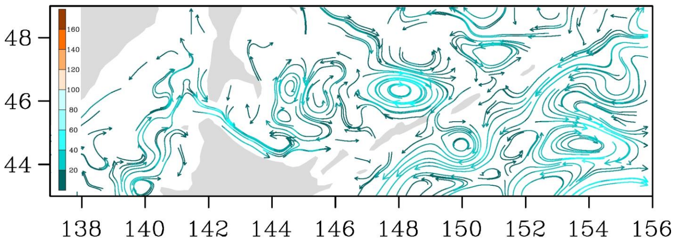
Рис. 3-9 Поверхностные течения, пролив Лаперуза, 25 июня 2020 г.
