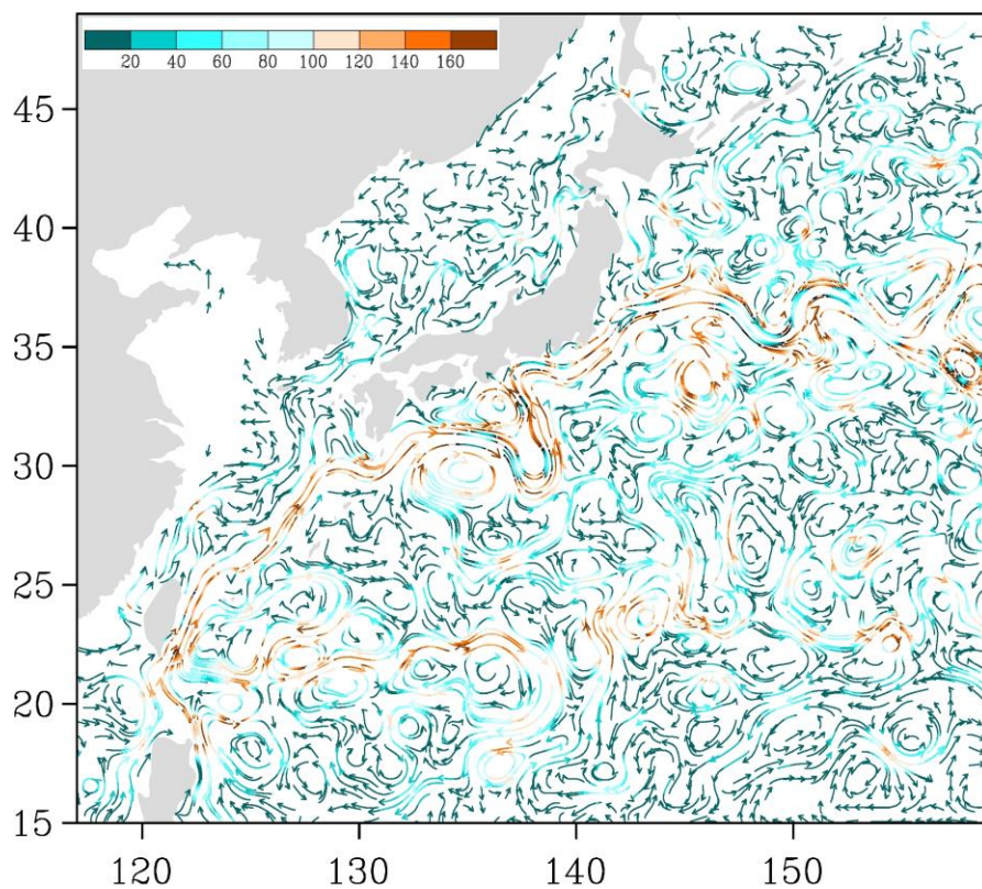
Рис. 3-5 Поверхностные течения западной части Тихого океана, 15 июня 2020 г.
