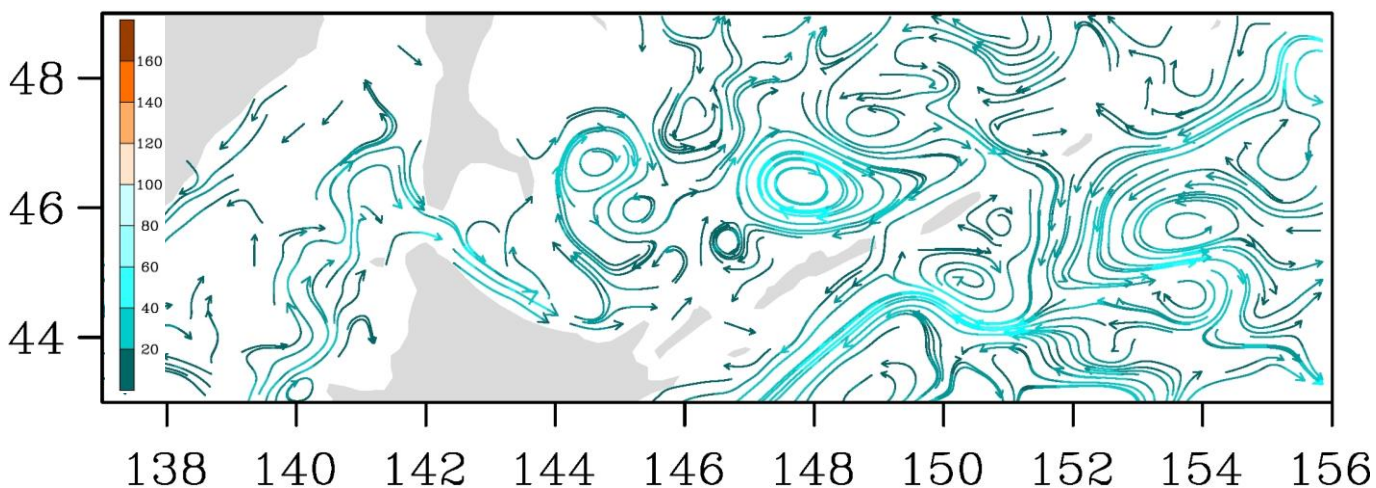
Рис. 3-7 Поверхностные течения, пролив Лаперуза, 5 июня 2020 г.
