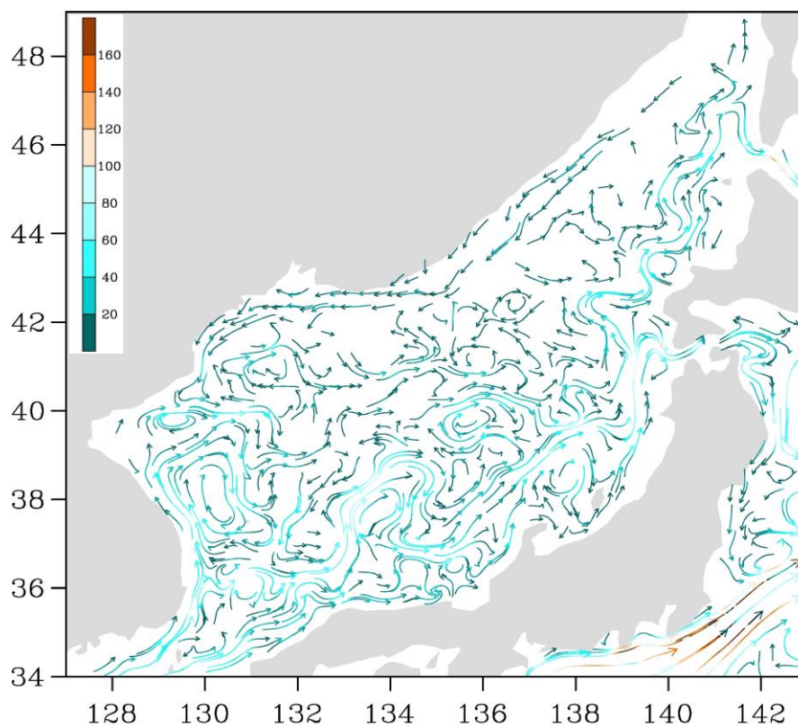
Рис. 3-3 Поверхностные течения Японского моря, 25 июня 2020 г.
