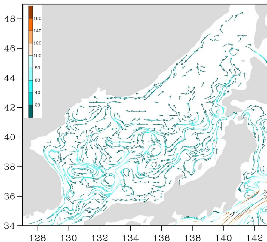
Рис. 3-3 Поверхностные течения Японского моря, 25 марта 2020 г.
