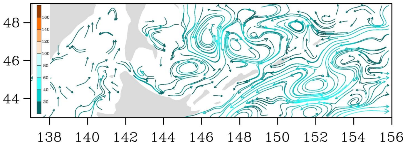
Рис. 3-8 Поверхностные течения, пролив Лаперуза, 15 марта 2020 г.
