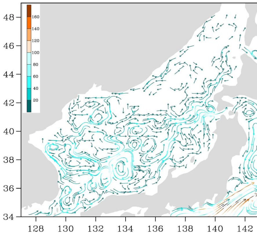
Рис. 3-2 Поверхностные течения Японского моря, 15 марта 2020 г.
