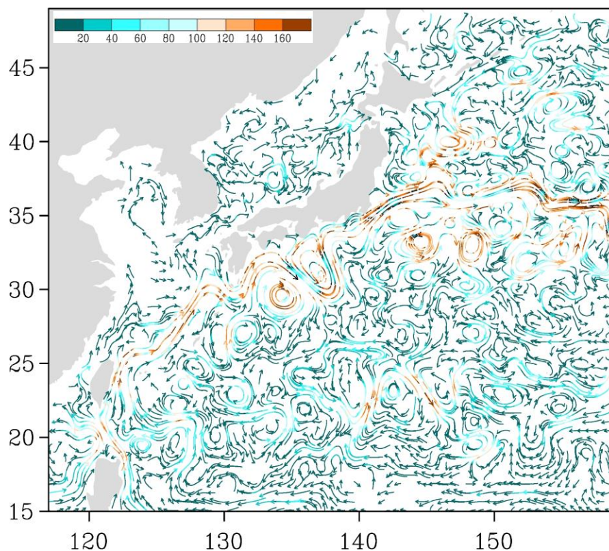
Рис. 3-5 Поверхностные течения западной части Тихого океана, 15 марта 2020 г.
