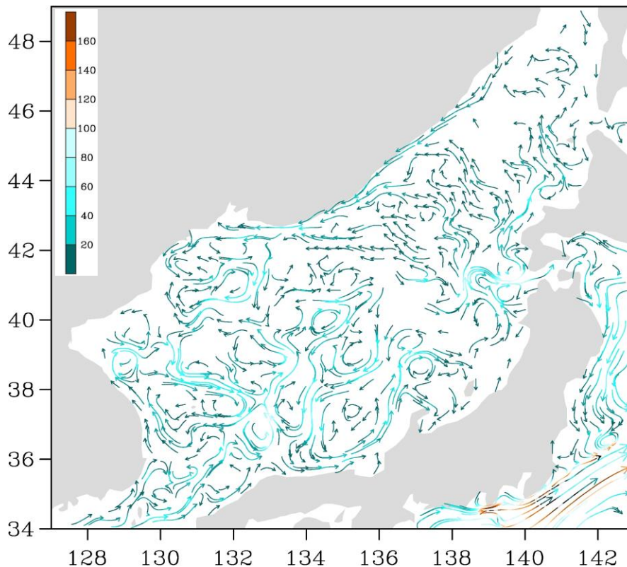
Рис. 3-1 Поверхностные течения Японского моря, 05 марта 2020 г.
