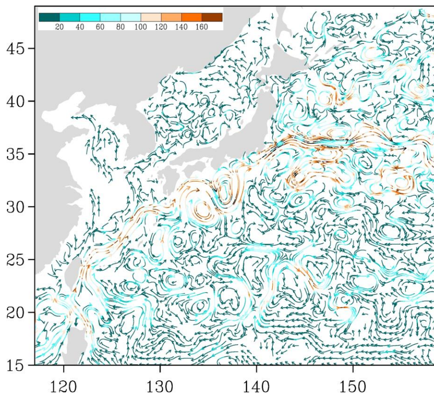
Рис. 3-4 Поверхностные течения западной части Тихого океана, 5 марта 2020 г.
