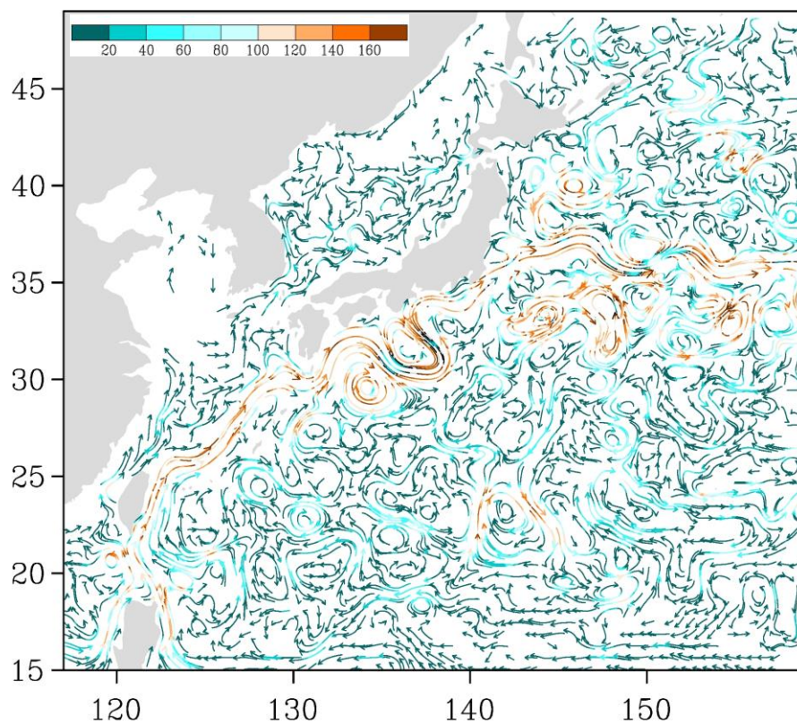
Рис. 3-6 Поверхностные течения западной части Тихого океана, 25 марта 2020 г.
