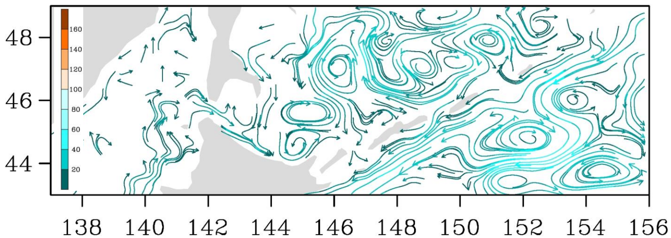
Рис. 3-9 Поверхностные течения, пролив Лаперуза, 25 марта 2020 г.
