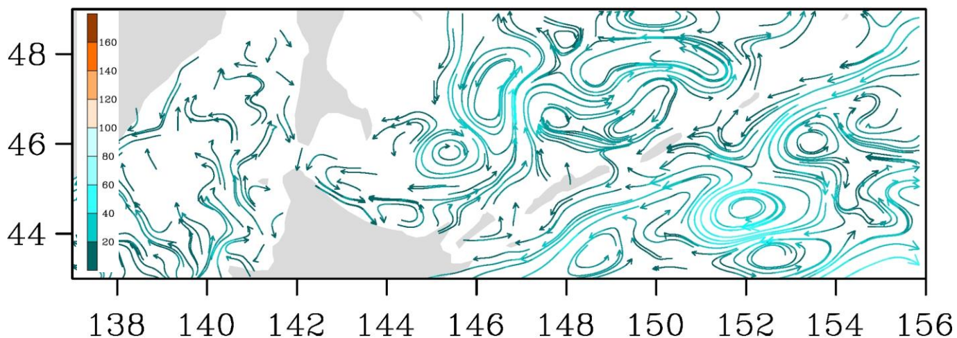
Рис. 3-7 Поверхностные течения, пролив Лаперуза, 5 марта 2020 г.
