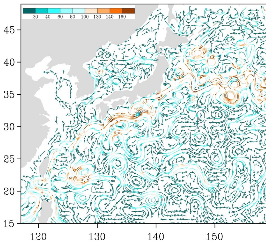
Рис. 3-6 Поверхностные течения западной части Тихого океана, 25 декабря 2020 г.
