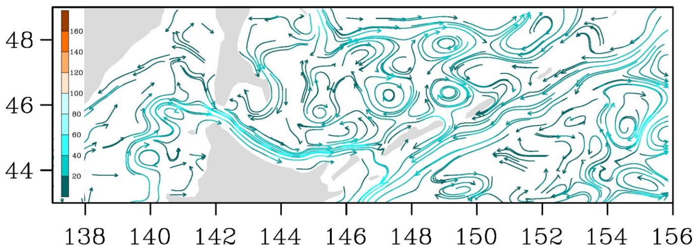
Рис. 3-9 Поверхностные течения, пролив Лаперуза, 25 декабря 2020 г.
