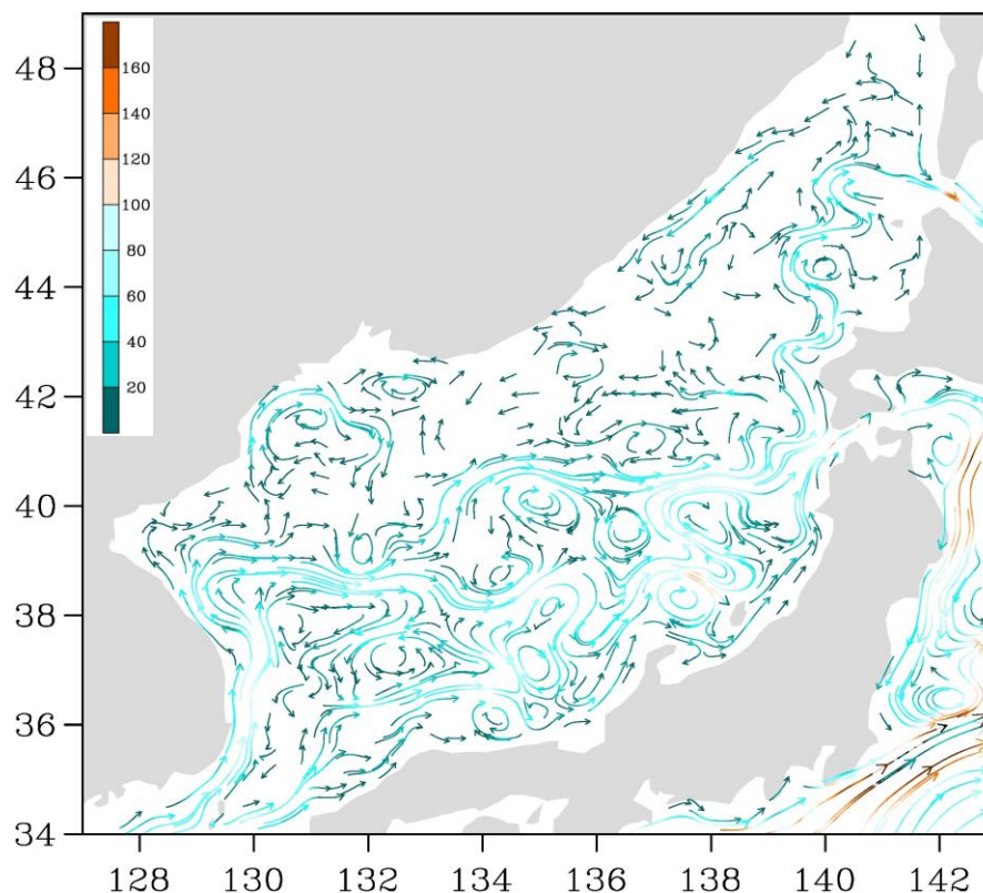
Рис. 3-1 Поверхностные течения Японского моря, 05 декабря 2020 г.
