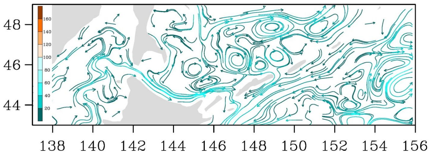
Рис. 3-8 Поверхностные течения, пролив Лаперуза, 15 декабря 2020 г.
