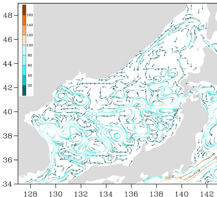
Рис. 3-3 Поверхностные течения Японского моря, 25 декабря 2020 г.
