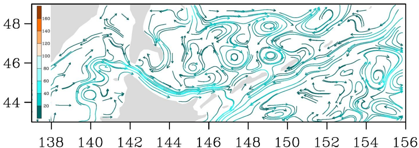
Рис. 3-7 Поверхностные течения, пролив Лаперуза, 5 декабря 2020 г.
