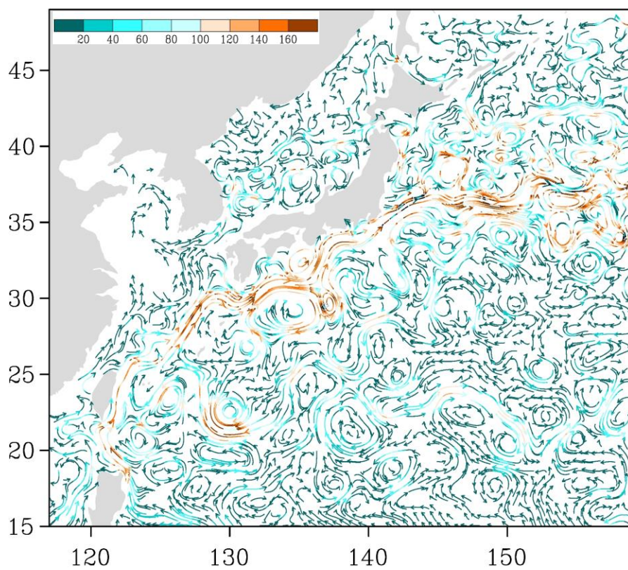
Рис. 3-6 Поверхностные течения западной части Тихого океана, 25 ноября 2020 г.
