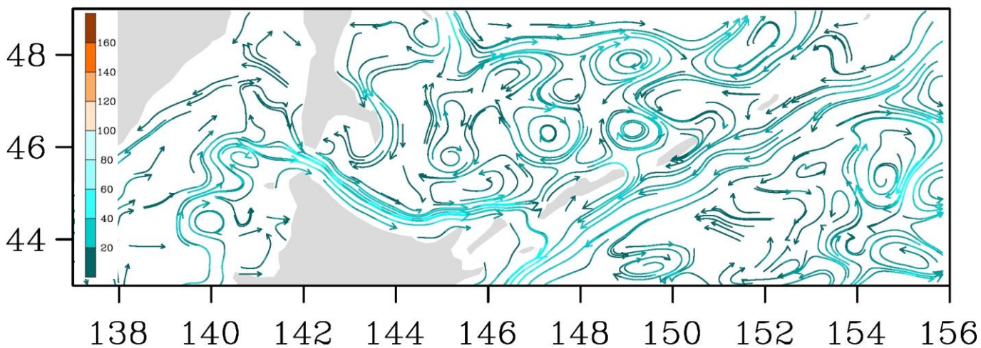
Рис. 3-9 Поверхностные течения, пролив Лаперуза, 25 ноября 2020 г.
