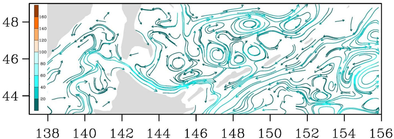
Рис. 3-8 Поверхностные течения, пролив Лаперуза, 15 ноября 2020 г.
