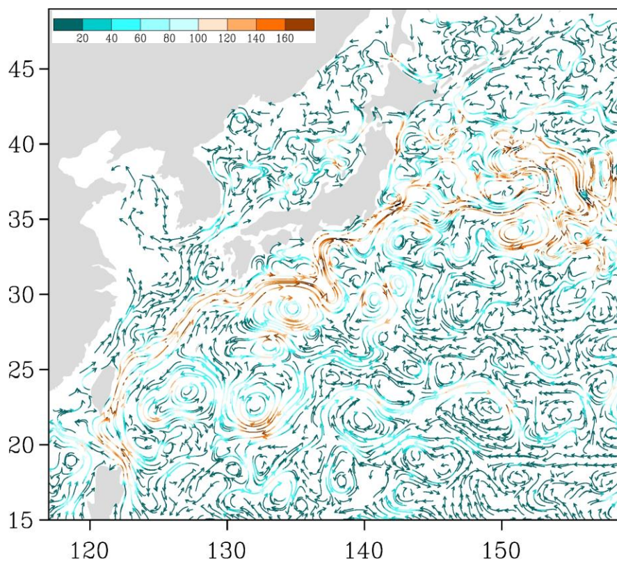
Рис. 3-4 Поверхностные течения западной части Тихого океана, 5 ноября 2020 г.
