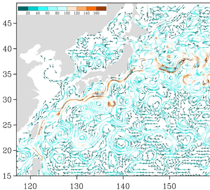
Рис. 3-5 Поверхностные течения западной части Тихого океана, 15 ноября 2020 г.
