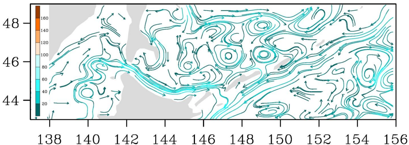
Рис. 3-7 Поверхностные течения, пролив Лаперуза, 5 ноября 2020 г.
