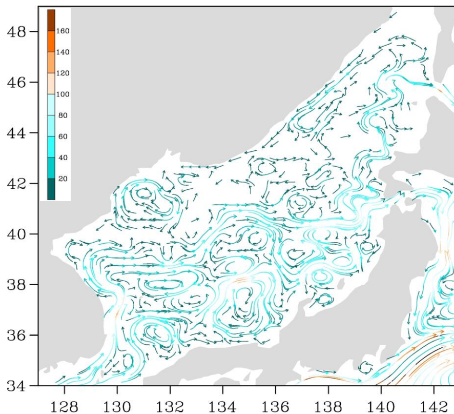
Рис. 3-2 Поверхностные течения Японского моря, 15 ноября 2020 г.
