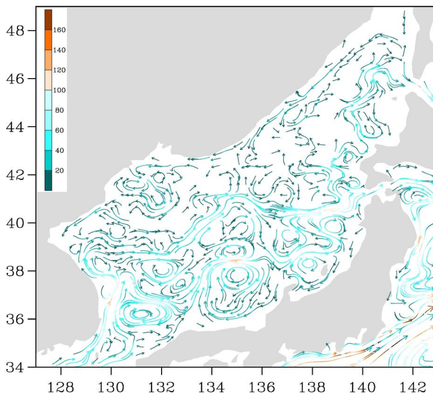
Рис. 3-3 Поверхностные течения Японского моря, 25 ноября 2020 г.
