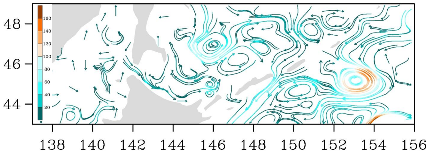
Рис. 3-8 Поверхностные течения, пролив Лаперуза, 15 января 2020 г.
