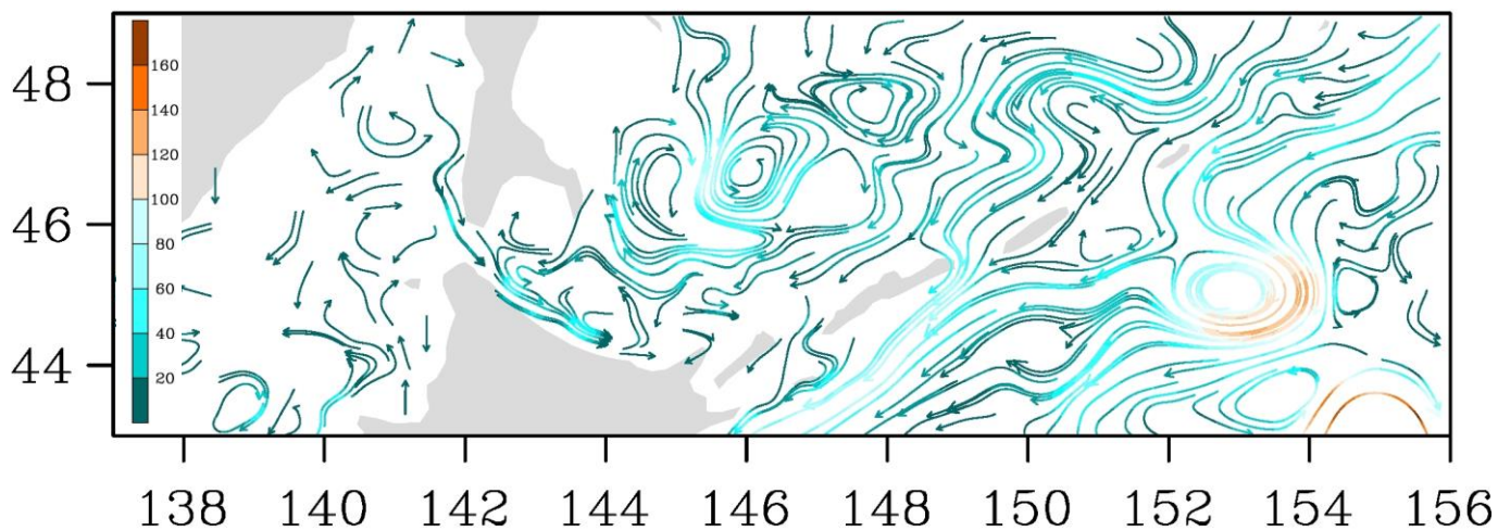
Рис. 3-9 Поверхностные течения, пролив Лаперуза, 25 января 2020 г.
