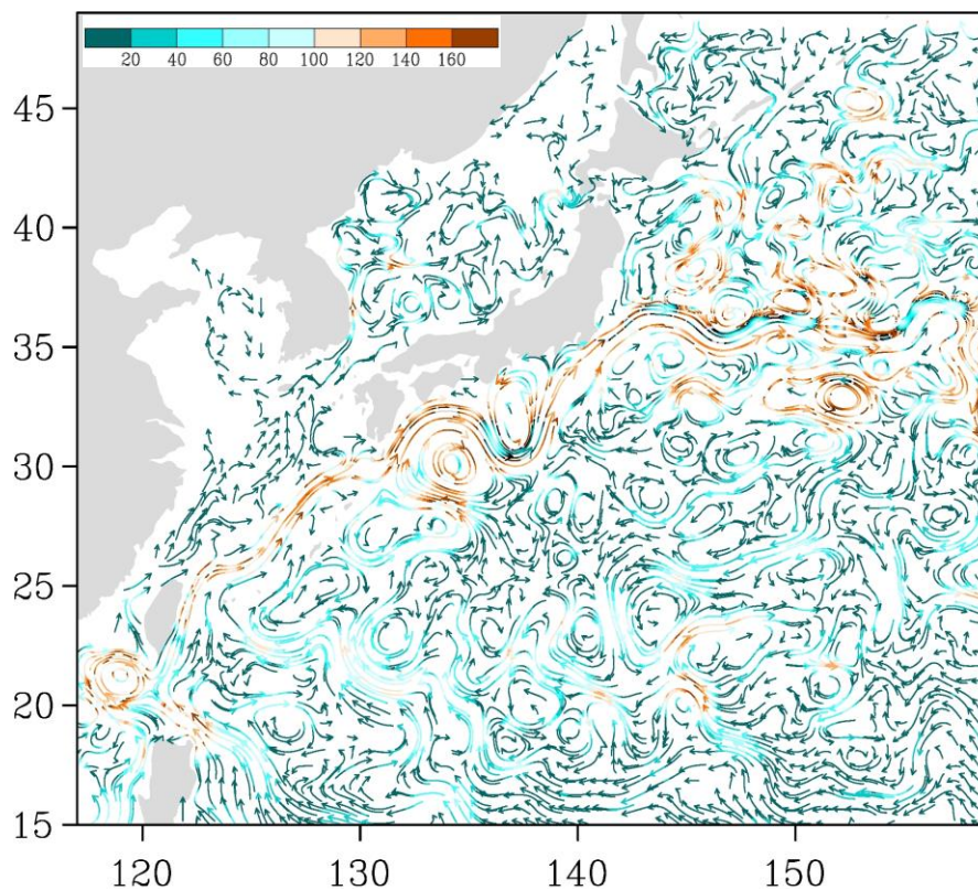
Рис. 3-4 Поверхностные течения западной части Тихого океана, 5 января 2020 г.
