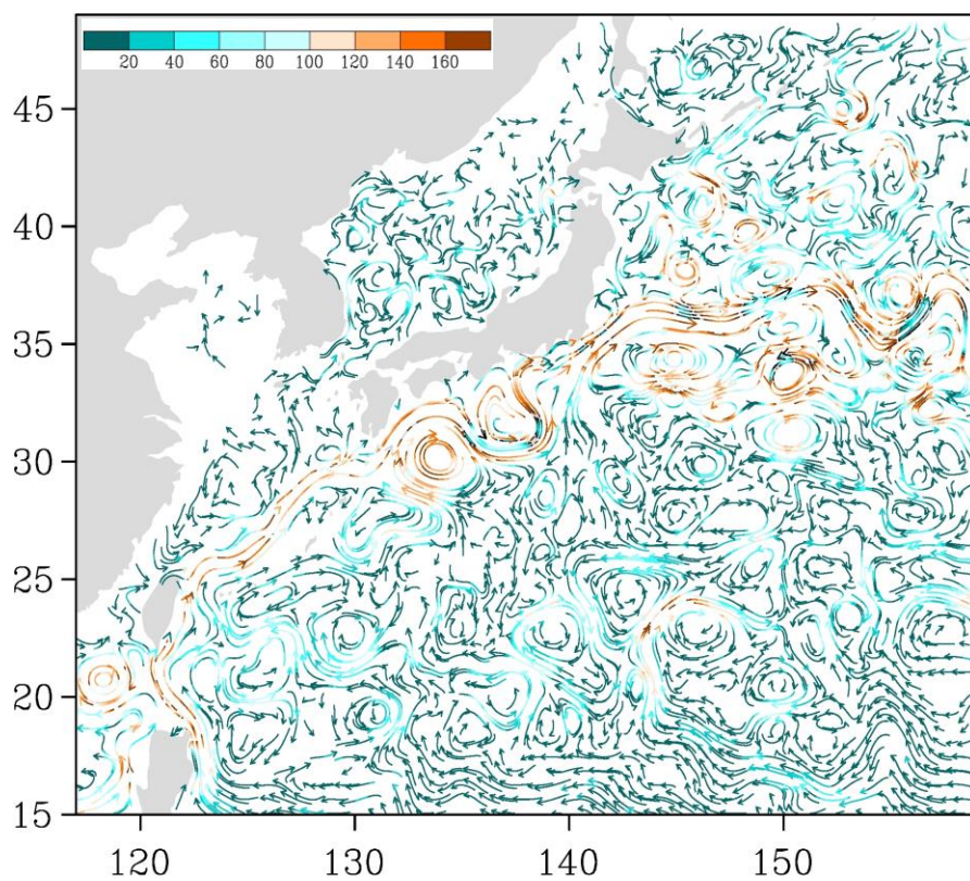
Рис. 3-6 Поверхностные течения западной части Тихого океана, 25 января 2020 г.
