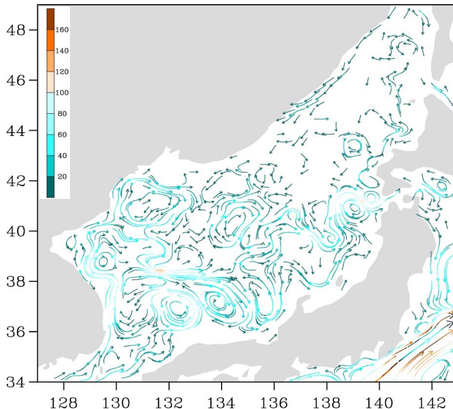
Рис. 3-1 Поверхностные течения Японского моря, 05 января 2020 г.
