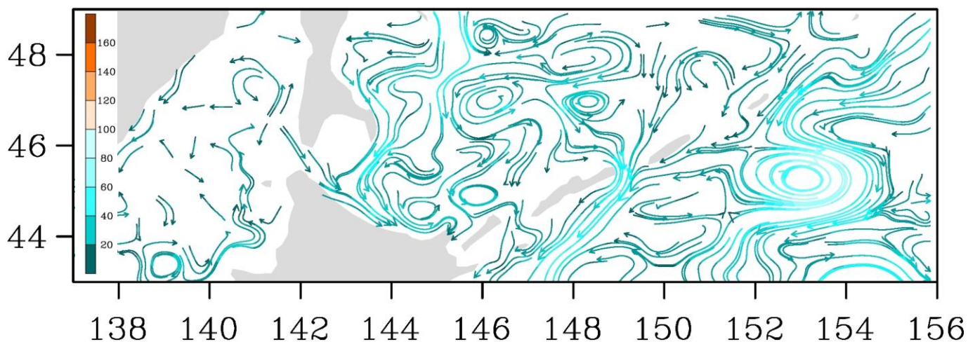
Рис. 3-7 Поверхностные течения, пролив Лаперуза, 5 января 2020 г.
