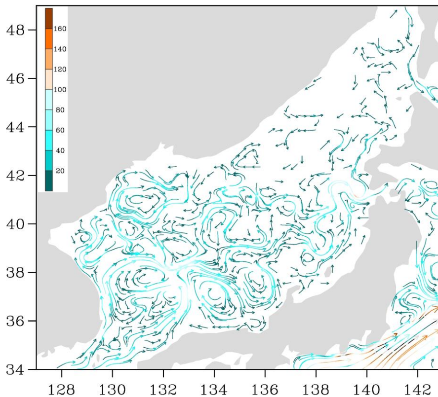
Рис. 3-3 Поверхностные течения Японского моря, 25 января 2020 г.
