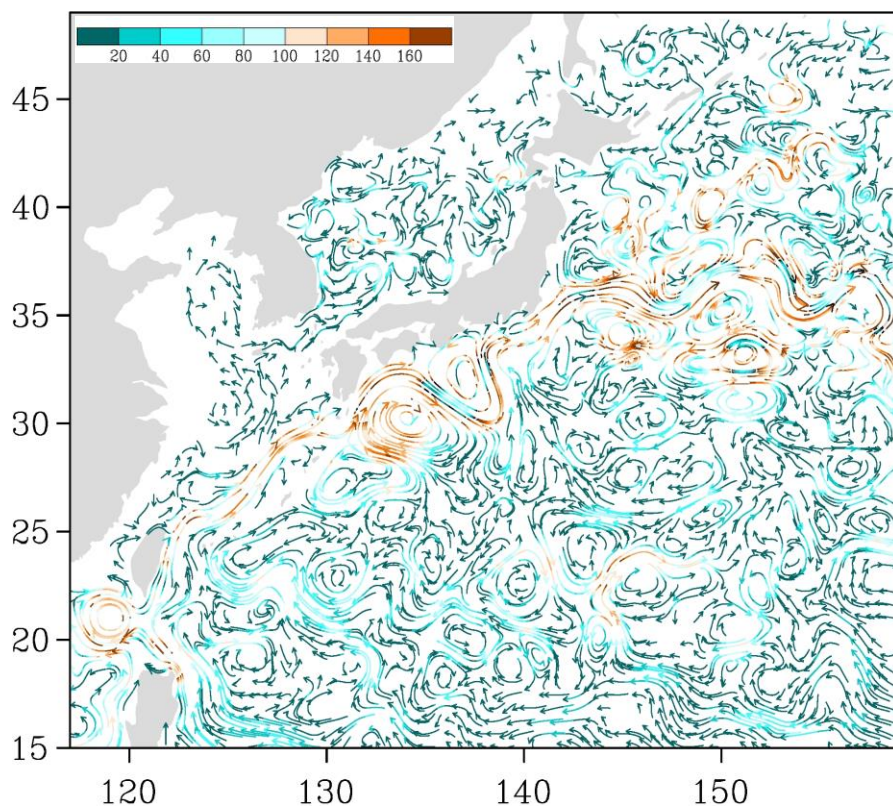
Рис. 3-5 Поверхностные течения западной части Тихого океана, 15 января 2020 г.
