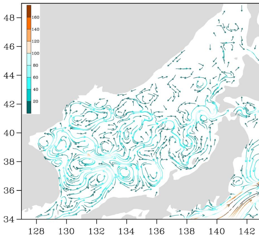
Рис. 3-2 Поверхностные течения Японского моря, 15 января 2020 г.
