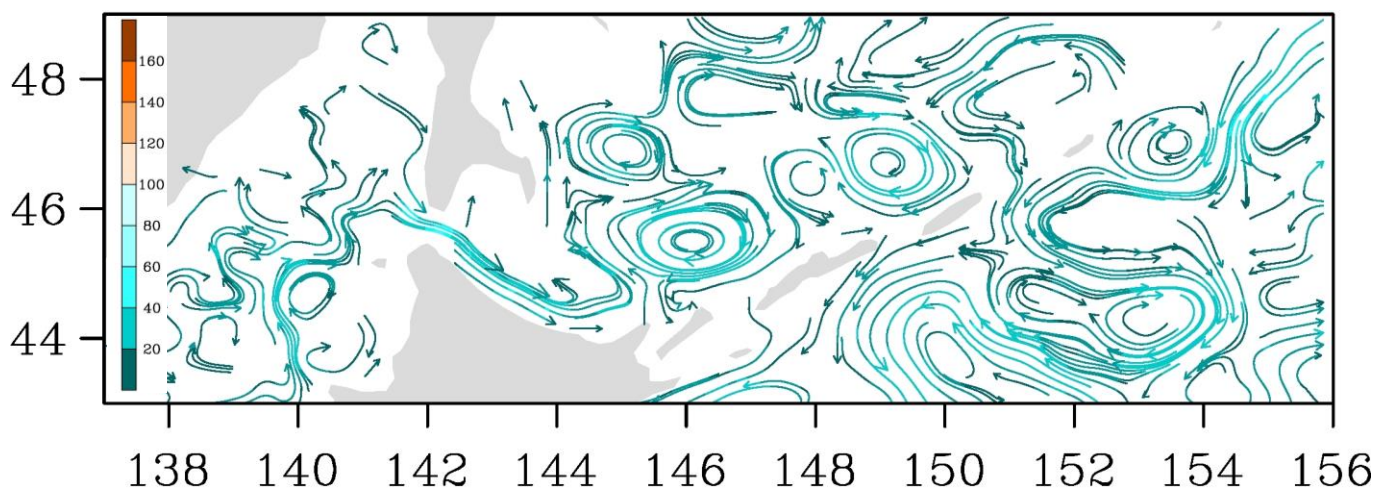
Рис. 3-8 Поверхностные течения, пролив Лаперуза, 15 августа 2017 г.
