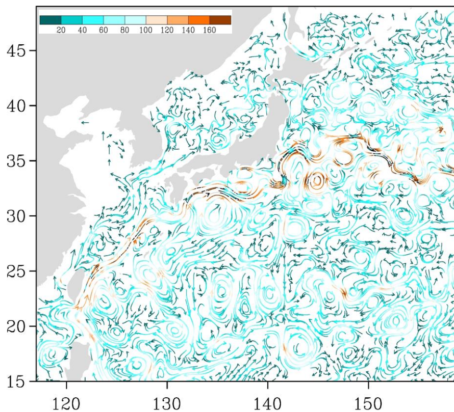
Рис. 3-6 Поверхностные течения западной части Тихого океана, 25 августа 2017 г.
