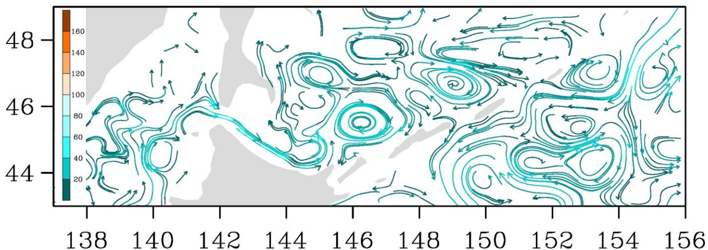
Рис. 3-7 Поверхностные течения, пролив Лаперуза, 5 августа 2017 г.
