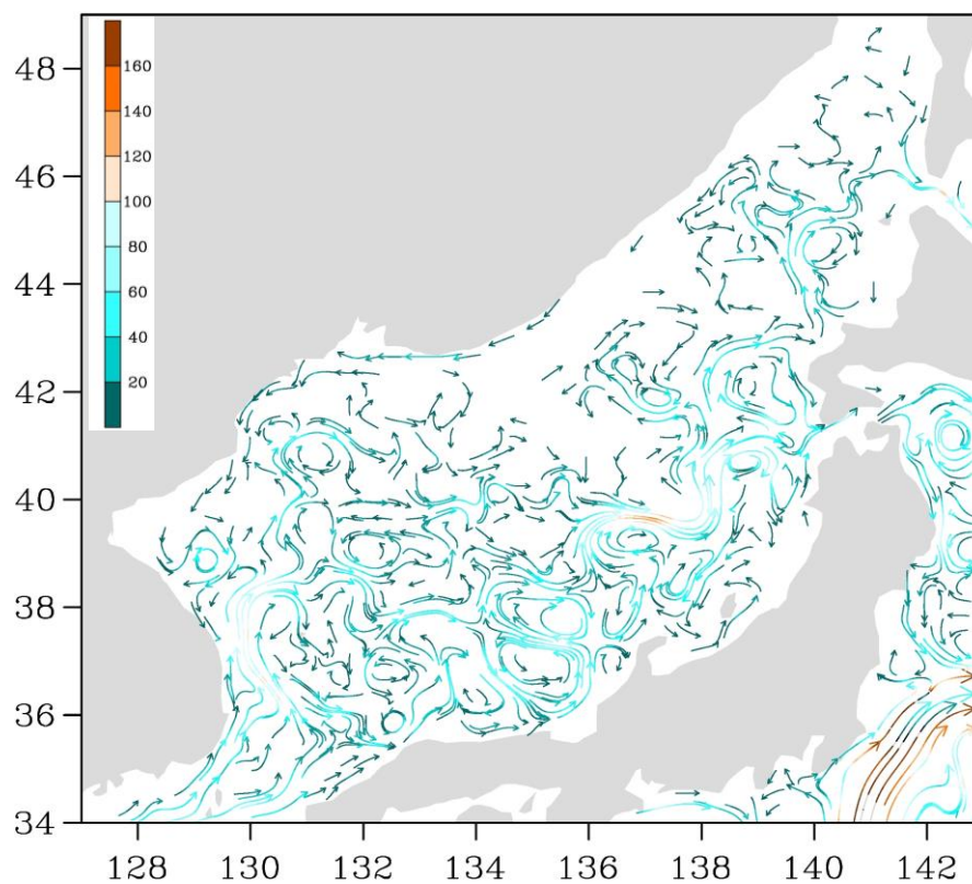
Рис. 3-2 Поверхностные течения Японского моря, 15 августа 2017 г.
