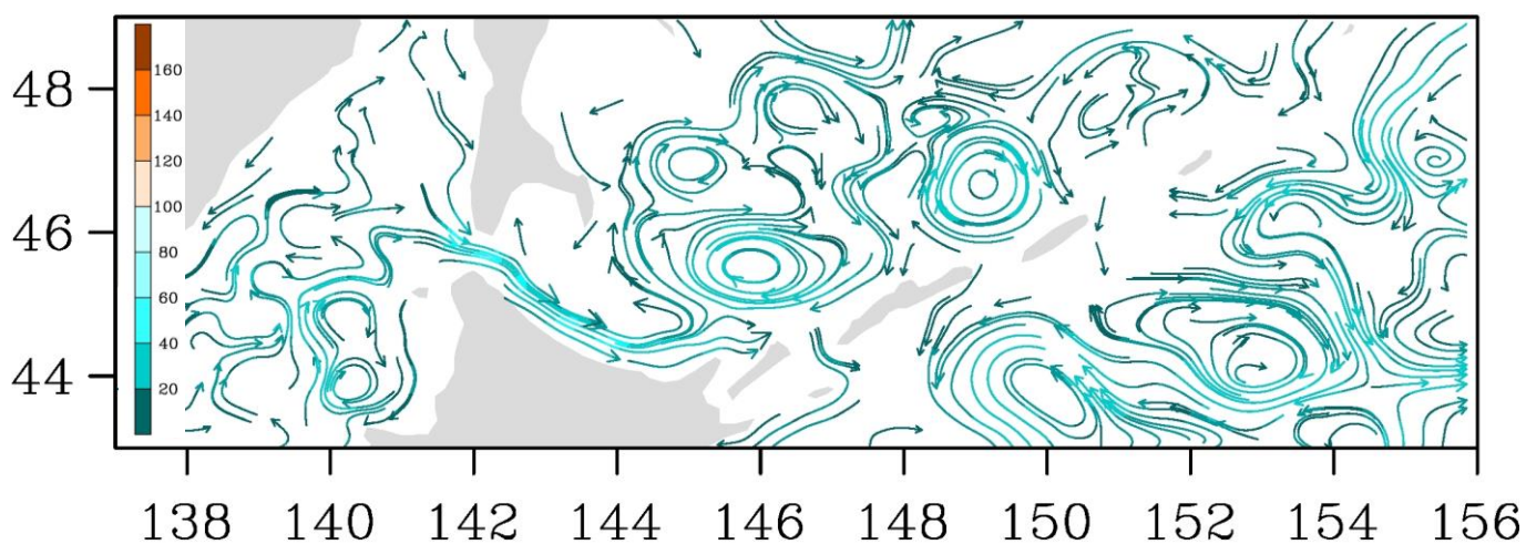
Рис. 3-9 Поверхностные течения, пролив Лаперуза, 25 августа 2017 г.
