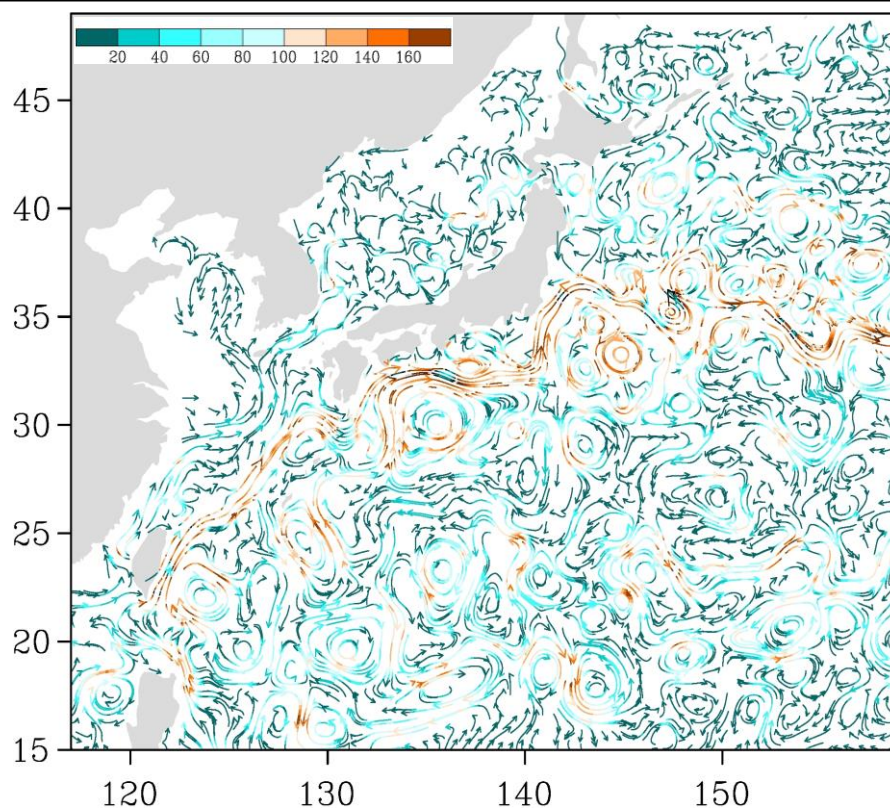
Рис. 3-5 Поверхностные течения западной части Тихого океана, 15 августа 2017 г.
