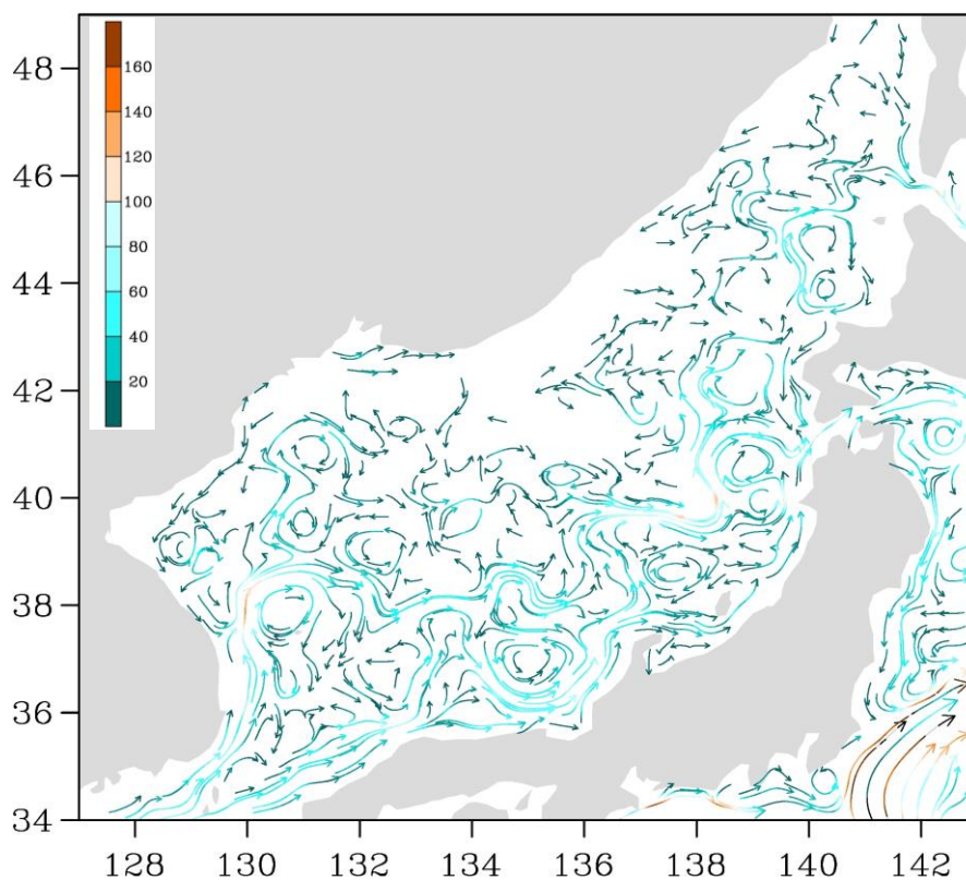
Рис. 3-3 Поверхностные течения Японского моря, 25 августа 2017 г.
