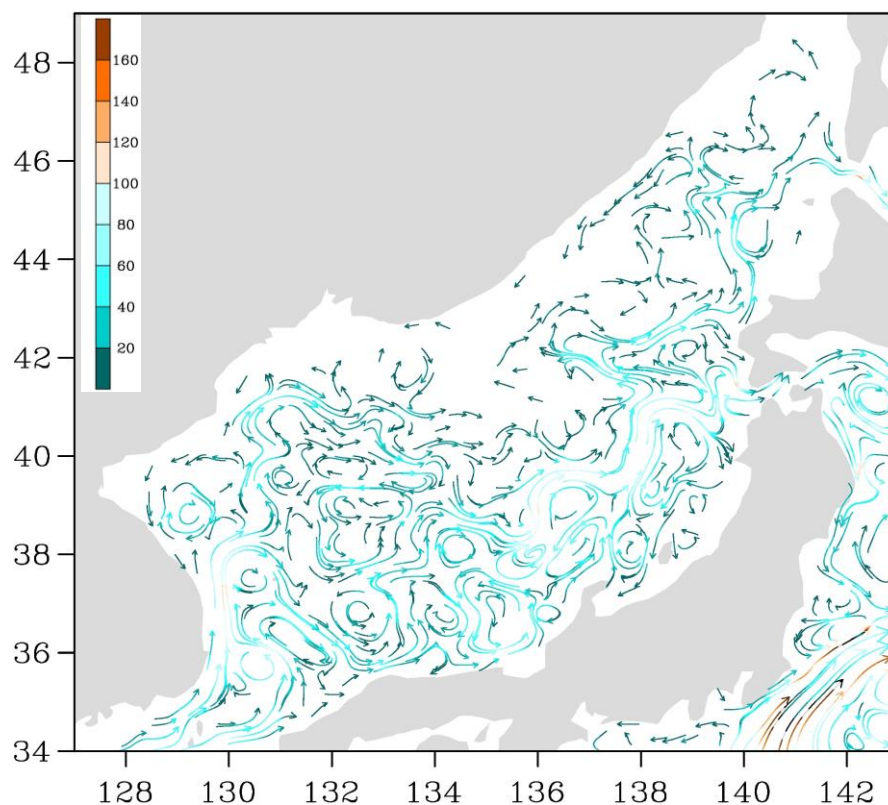
Рис. 3-1 Поверхностные течения Японского моря, 05 августа 2017 г.
