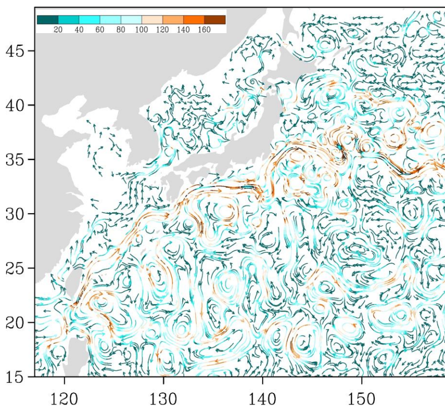
Рис. 3-4 Поверхностные течения западной части Тихого океана, 5 августа 2017 г.
