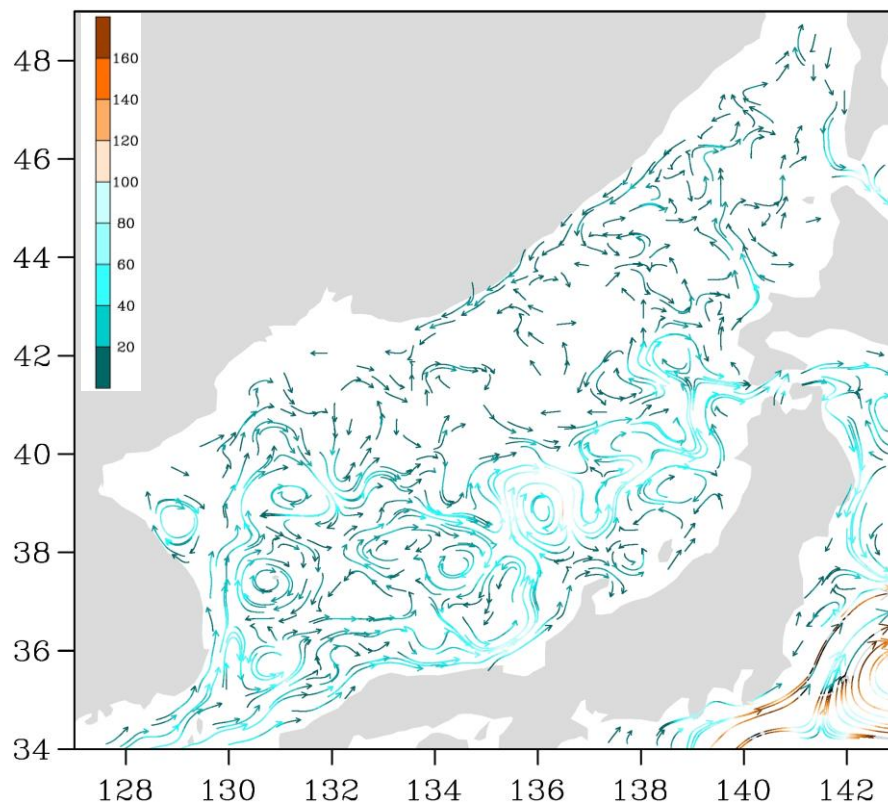
Рис. 3-2 Поверхностные течения Японского моря, 15 июня 2017 г.
