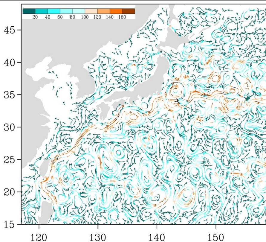
Рис. 3-5 Поверхностные течения западной части Тихого океана, 15 июня 2017 г.
