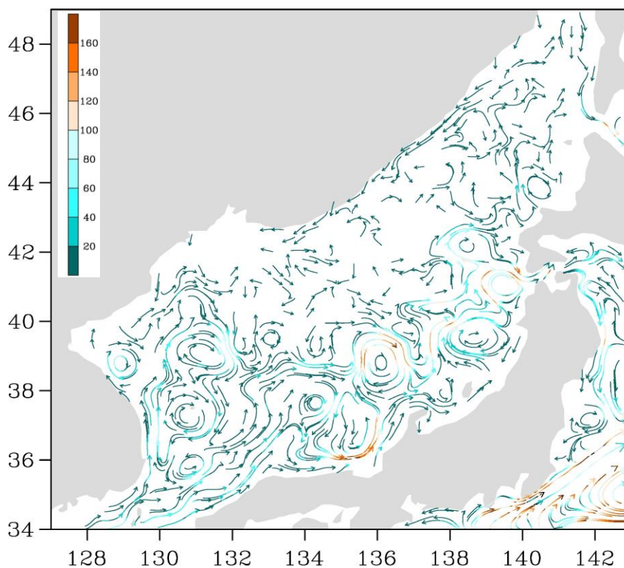
Рис. 3-3 Поверхностные течения Японского моря, 25 июня 2017 г.
