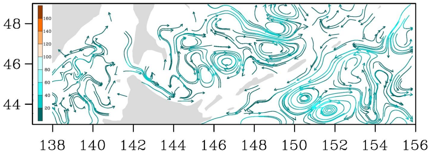
Рис. 3-7 Поверхностные течения, пролив Лаперуза, 5 июня 2017 г.
