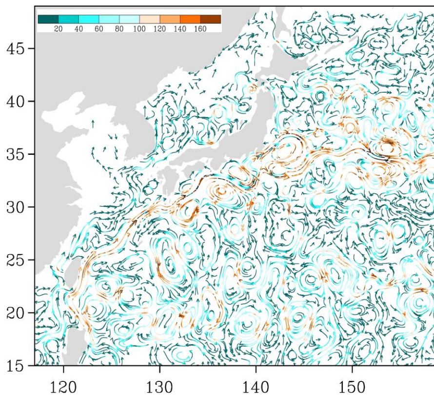
Рис. 3-6 Поверхностные течения западной части Тихого океана, 25 июня 2017 г.
