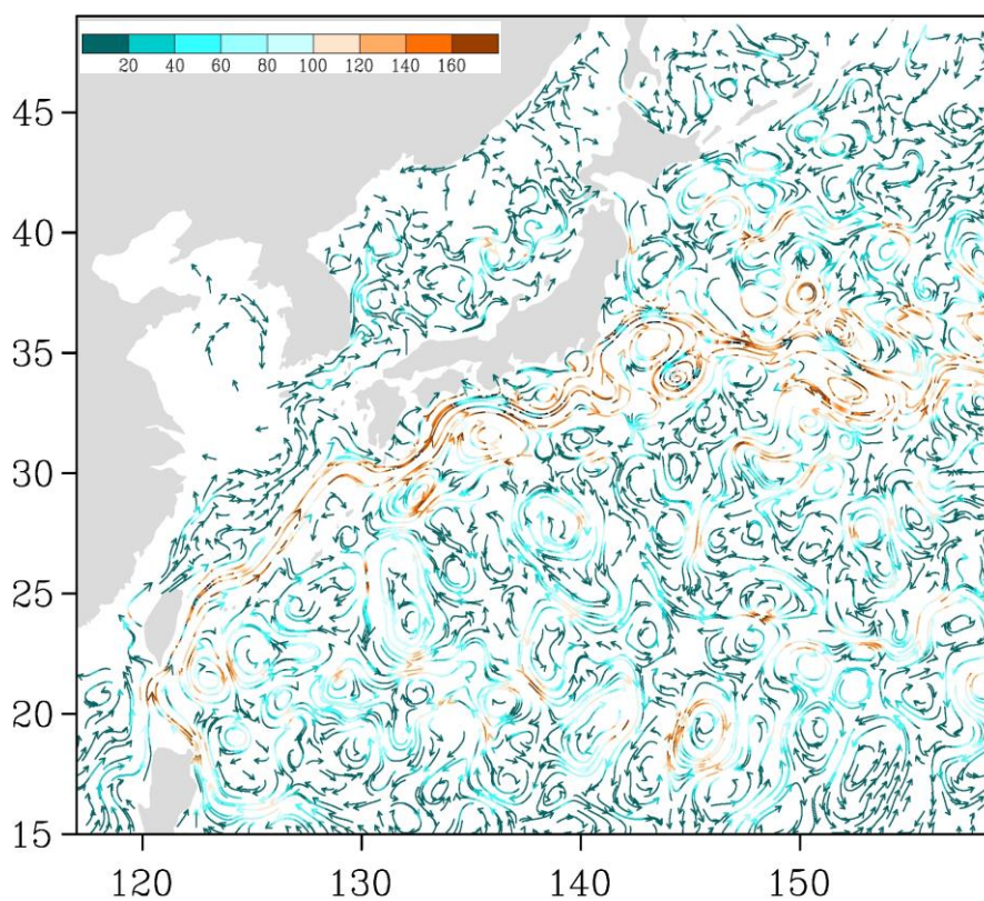
Рис. 3-4 Поверхностные течения западной части Тихого океана, 5 июня 2017 г.
