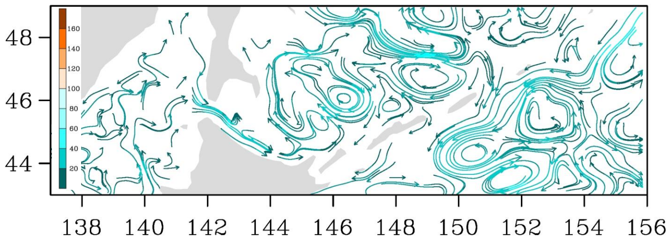
Рис. 3-8 Поверхностные течения, пролив Лаперуза, 15 июня 2017 г.
