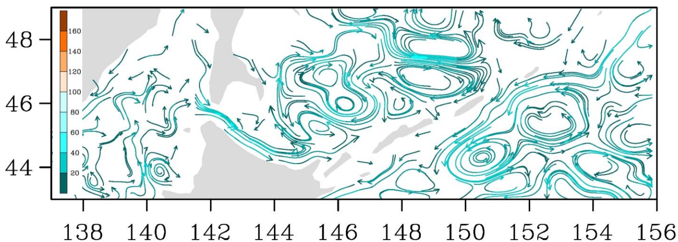
Рис. 3-9 Поверхностные течения, пролив Лаперуза, 25 июня 2017 г.
