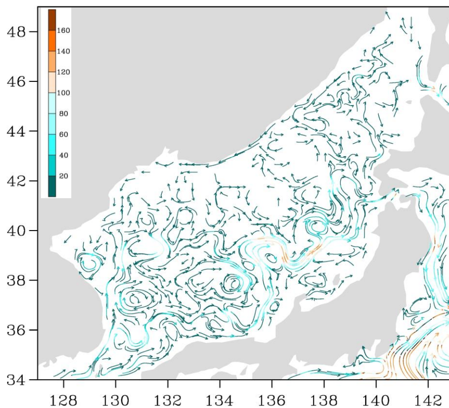
Рис. 3-1 Поверхностные течения Японского моря, 05 июня 2017 г.
