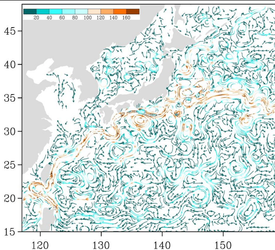
Рис. 3-5 Поверхностные течения западной части Тихого океана, 15 марта 2017 г.
