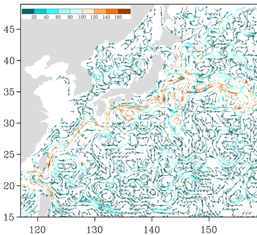
Рис. 3-4 Поверхностные течения западной части Тихого океана, 5 марта 2017 г.
