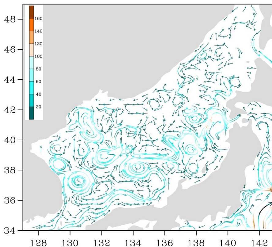
Рис. 3-1 Поверхностные течения Японского моря, 05 марта 2017 г.
