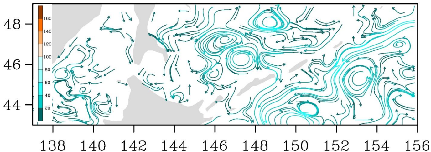
Рис. 3-8 Поверхностные течения, пролив Лаперуза, 15 марта 2017 г.
