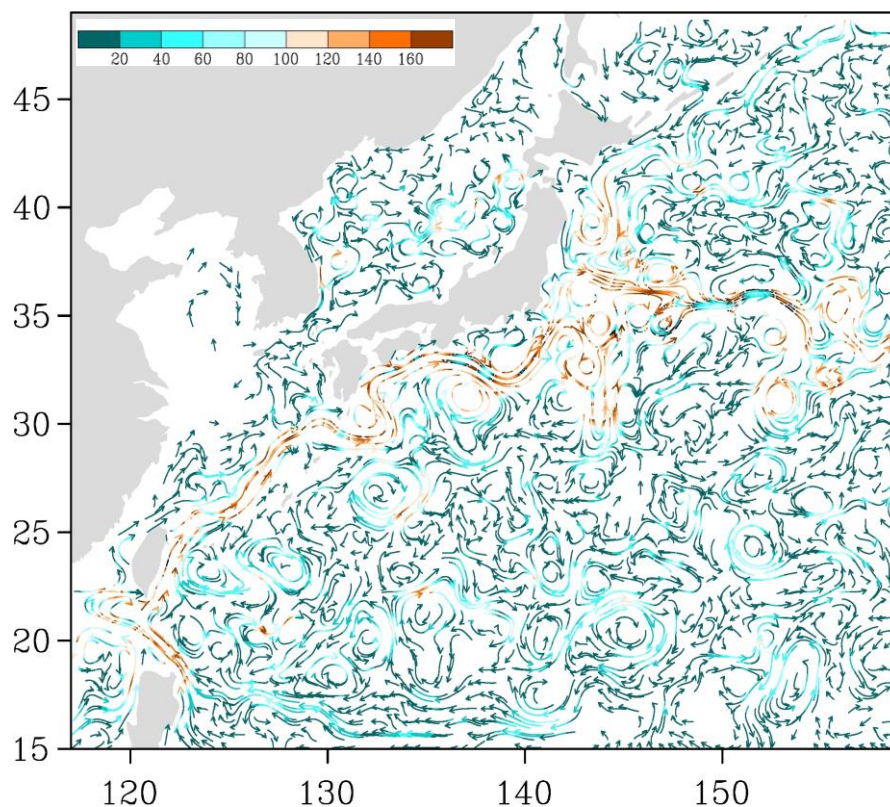
Рис. 3-6 Поверхностные течения западной части Тихого океана, 25 марта 2017 г.
