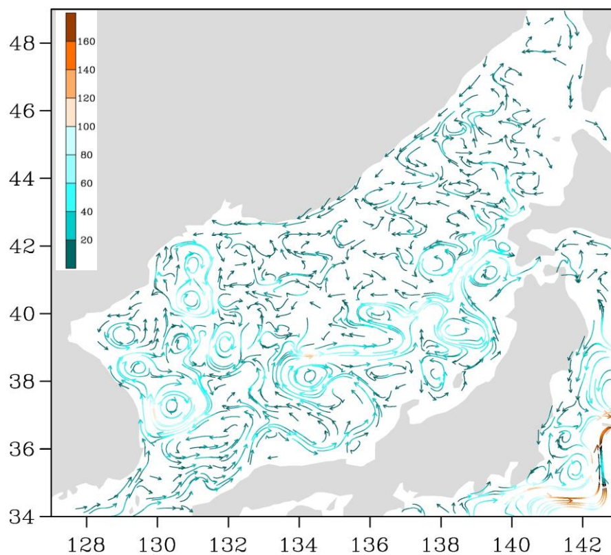
Рис. 3-2 Поверхностные течения Японского моря, 15 марта 2017 г.
