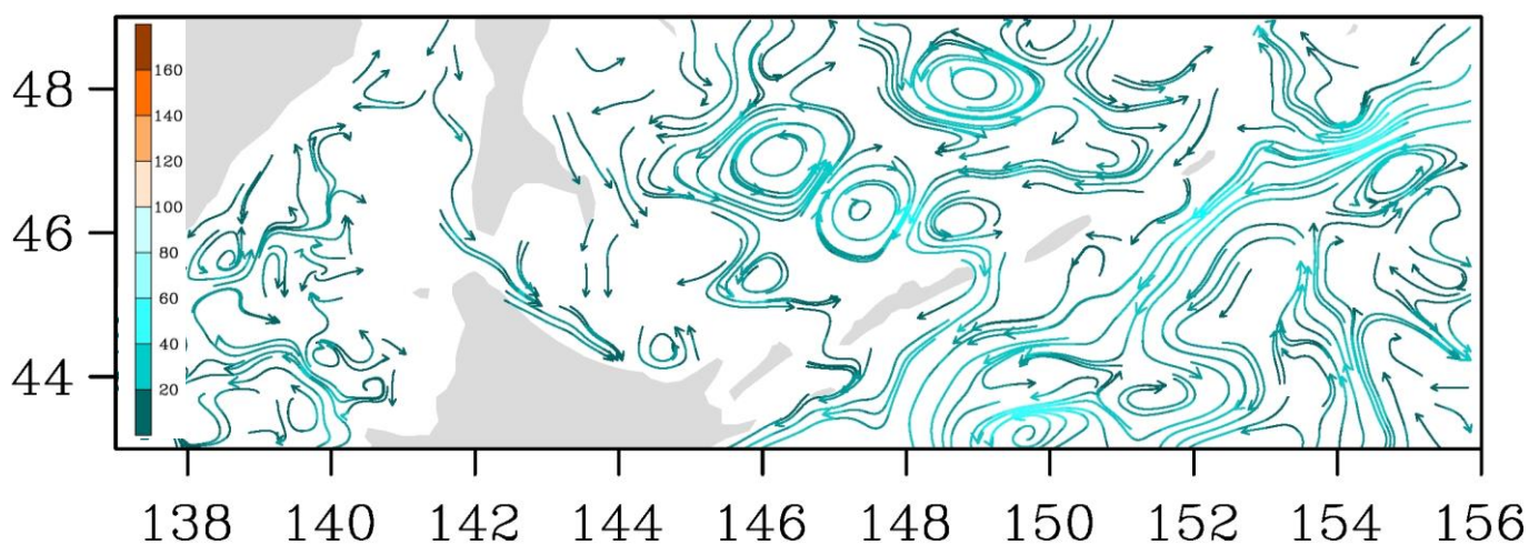
Рис. 3-9 Поверхностные течения, пролив Лаперуза, 25 марта 2017 г.
