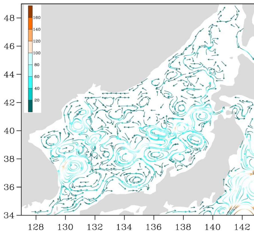
Рис. 3-3 Поверхностные течения Японского моря, 25 марта 2017 г.
