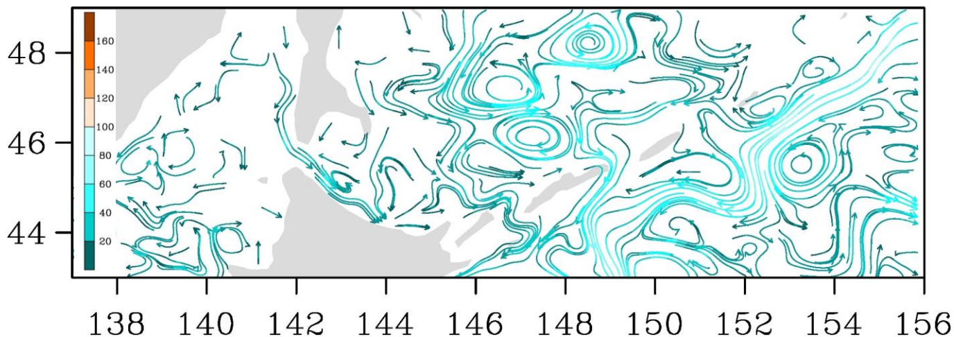
Рис. 3-7 Поверхностные течения, пролив Лаперуза, 5 марта 2017 г.
