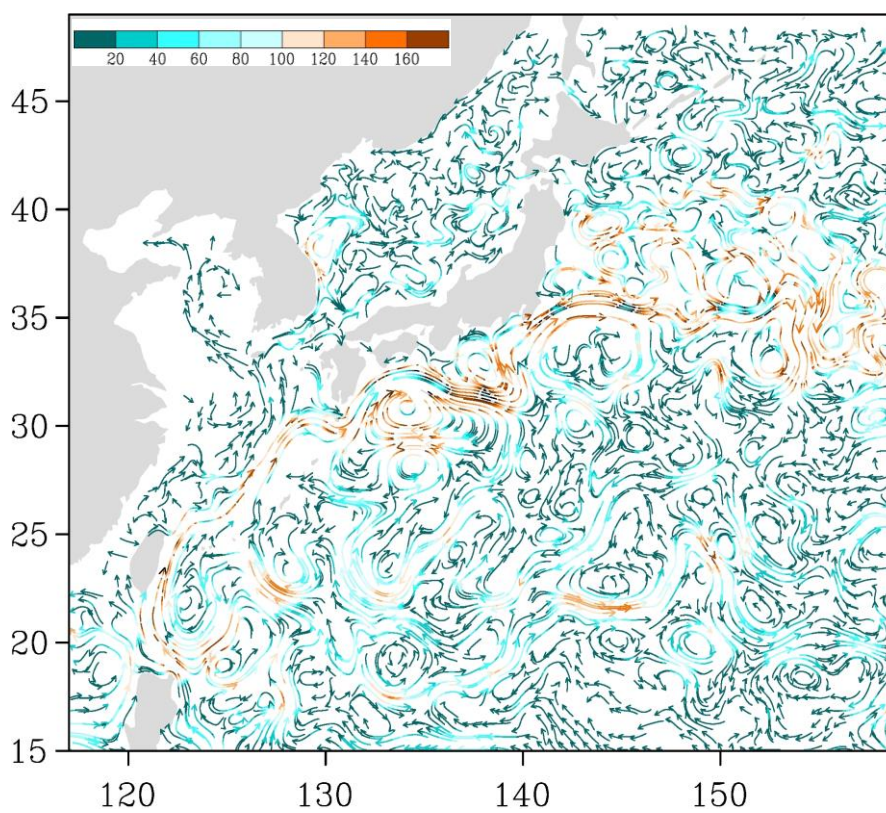
Рис. 3-4 Поверхностные течения западной части Тихого океана, 5 декабря 2017 г.
