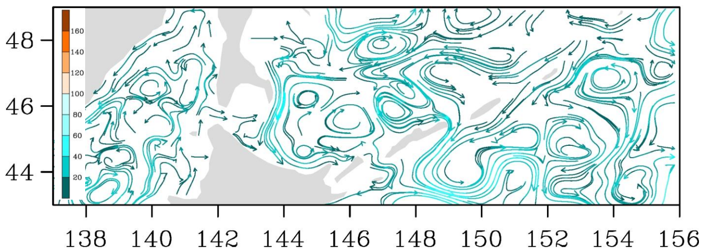
Рис. 3-8 Поверхностные течения, пролив Лаперуза, 15 декабря 2017 г.
