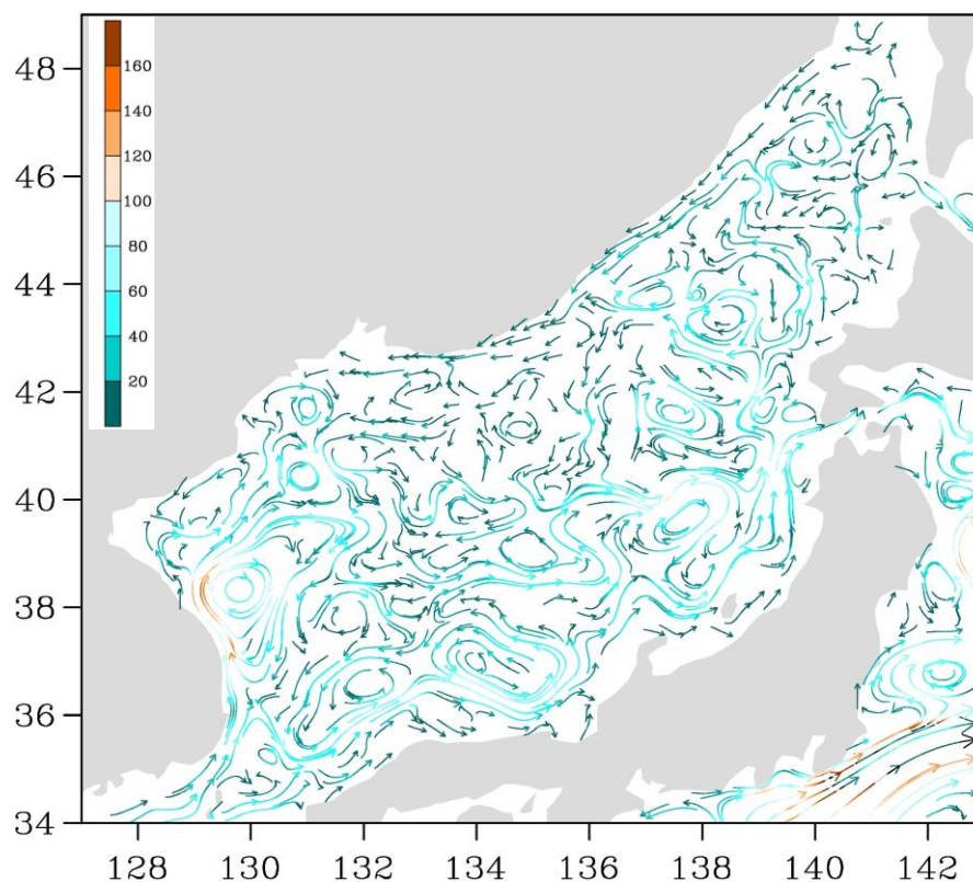
Рис. 3-1 Поверхностные течения Японского моря, 05 декабря 2017 г.
