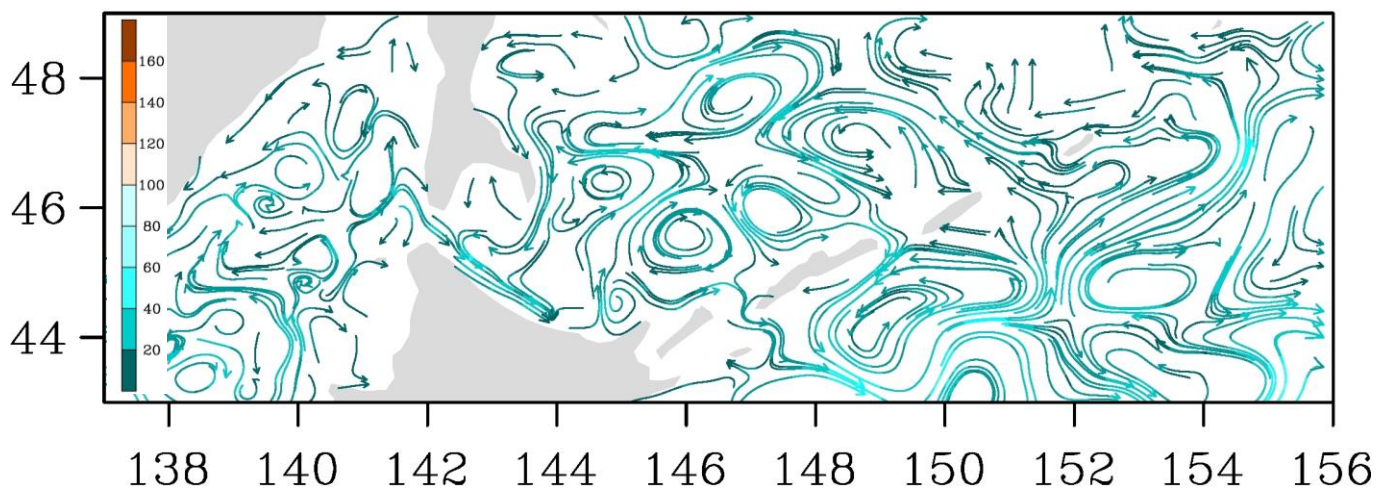
Рис. 3-7 Поверхностные течения, пролив Лаперуза, 5 декабря 2017 г.
