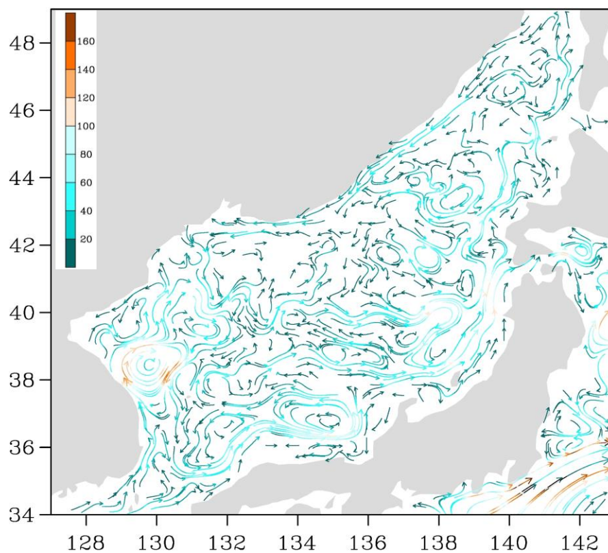
Рис. 3-2 Поверхностные течения Японского моря, 15 декабря 2017 г.
