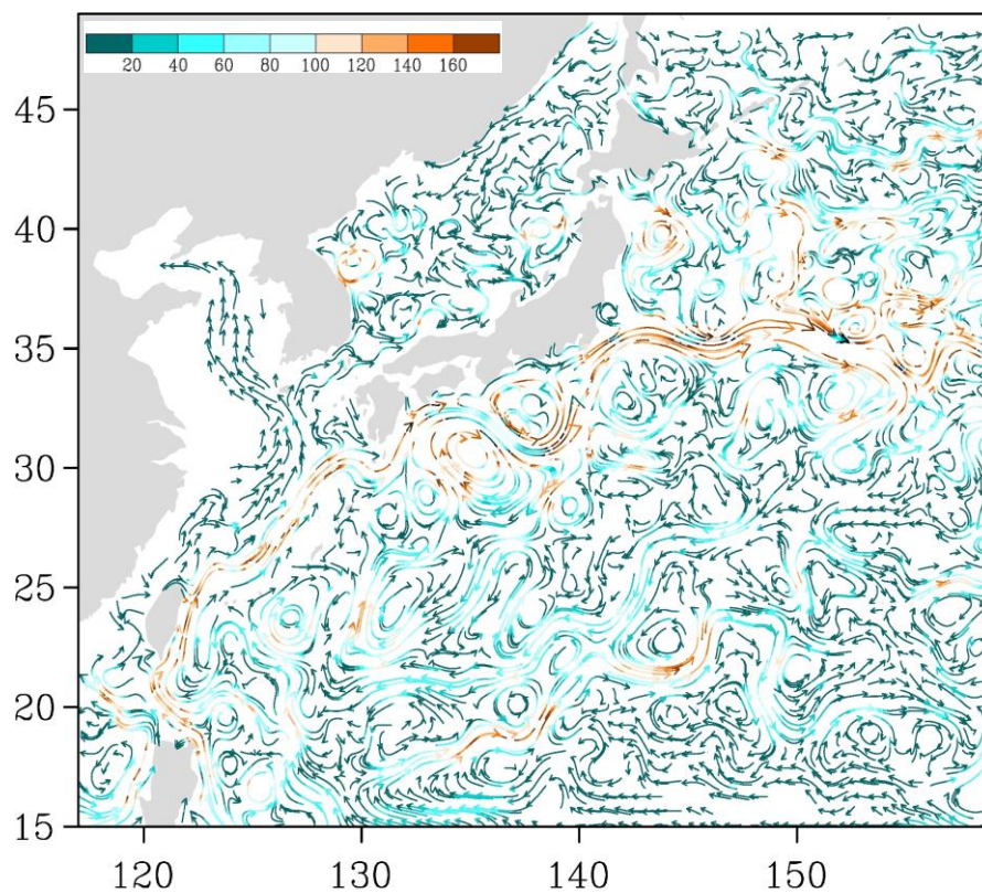
Рис. 3-6 Поверхностные течения западной части Тихого океана, 25 декабря 2017 г.
