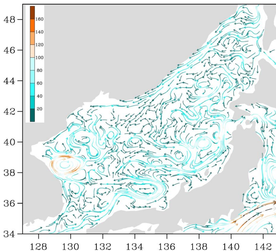
Рис. 3-3 Поверхностные течения Японского моря, 25 декабря 2017 г.
