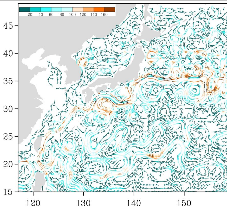
Рис. 3-5 Поверхностные течения западной части Тихого океана, 15 декабря 2017 г.
